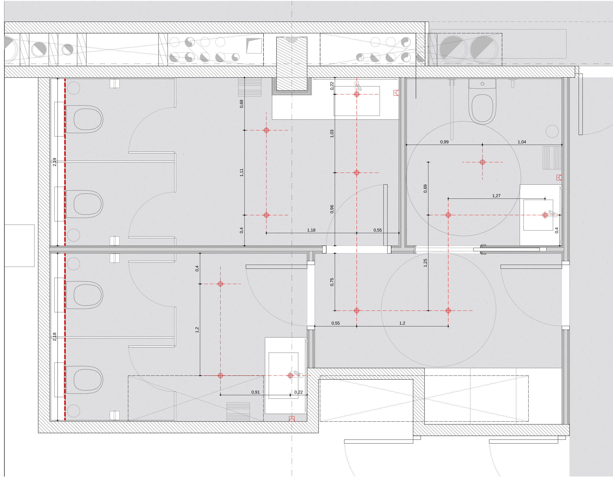
E5 Planta Il·luminació Banyes Comuns P00 A1 1:25 A3 1:50 0 25 50 75 100 150 200 250 cm
