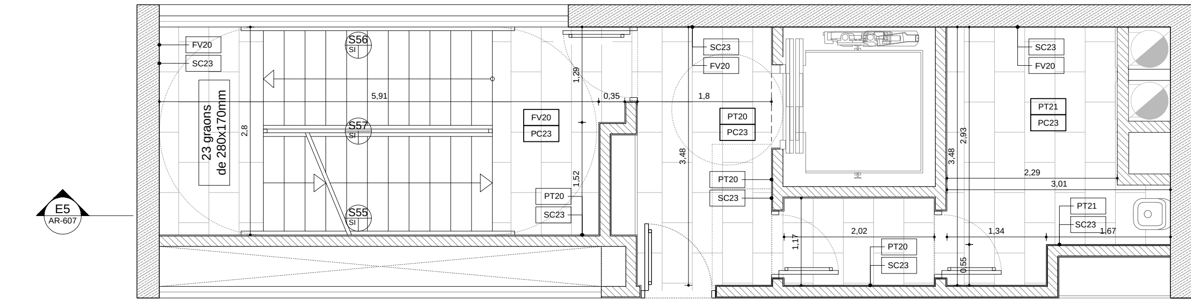
A5 Planta escala - P01
