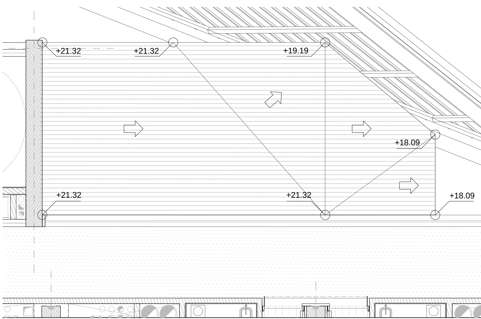
F5 Planta coberta
