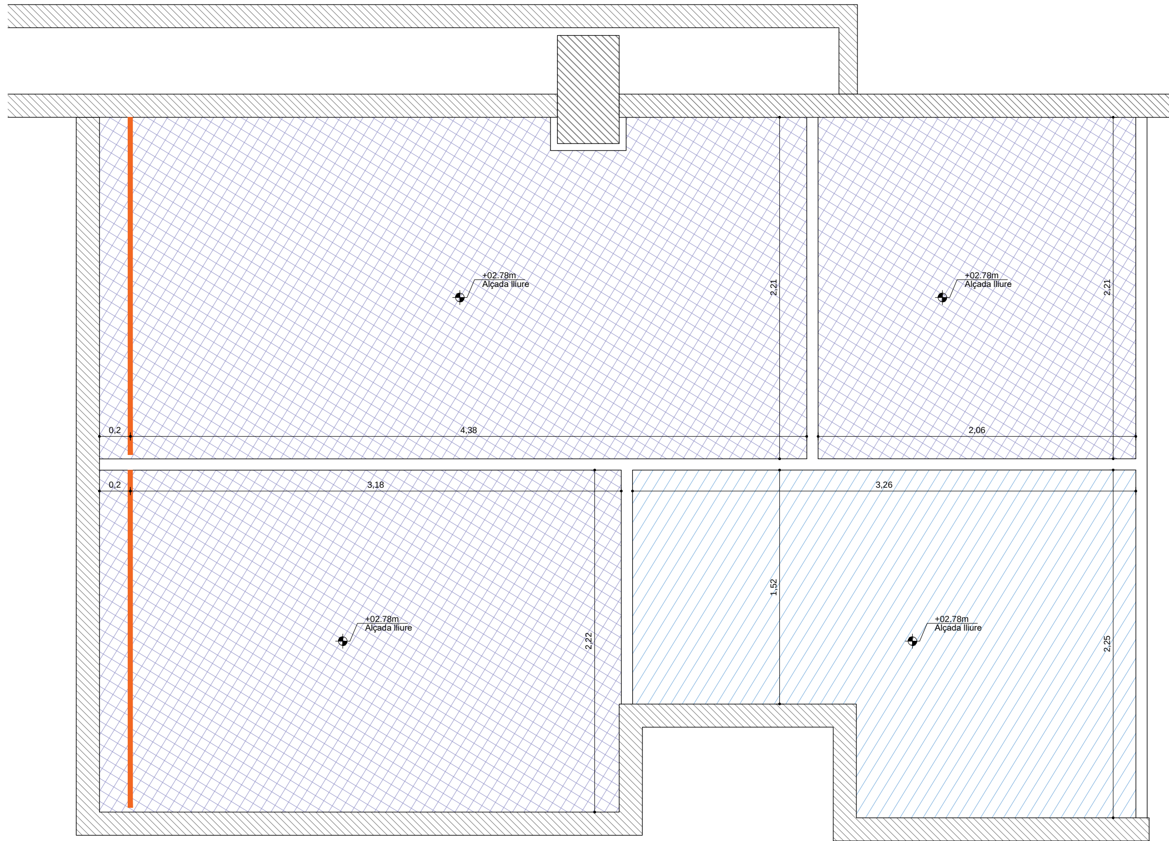
A5 Planta Fals Sostre Banyes Comuns P01 A1 1:25 A3 1:50 0 25 50 75 100 150 200 250 cm
