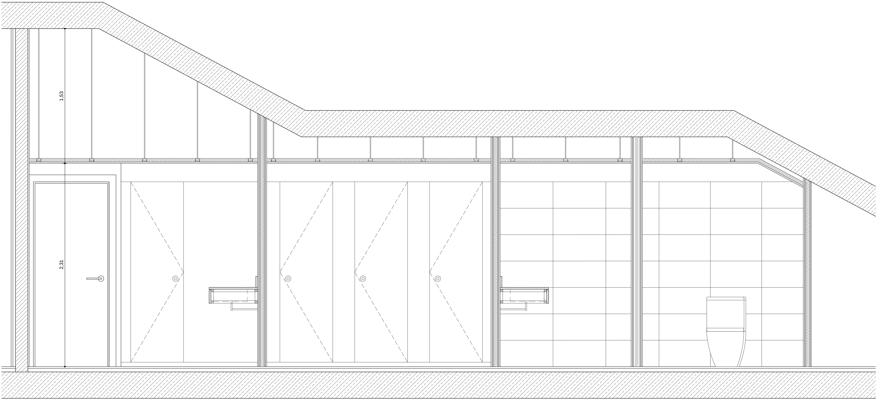
A6 Secció A
