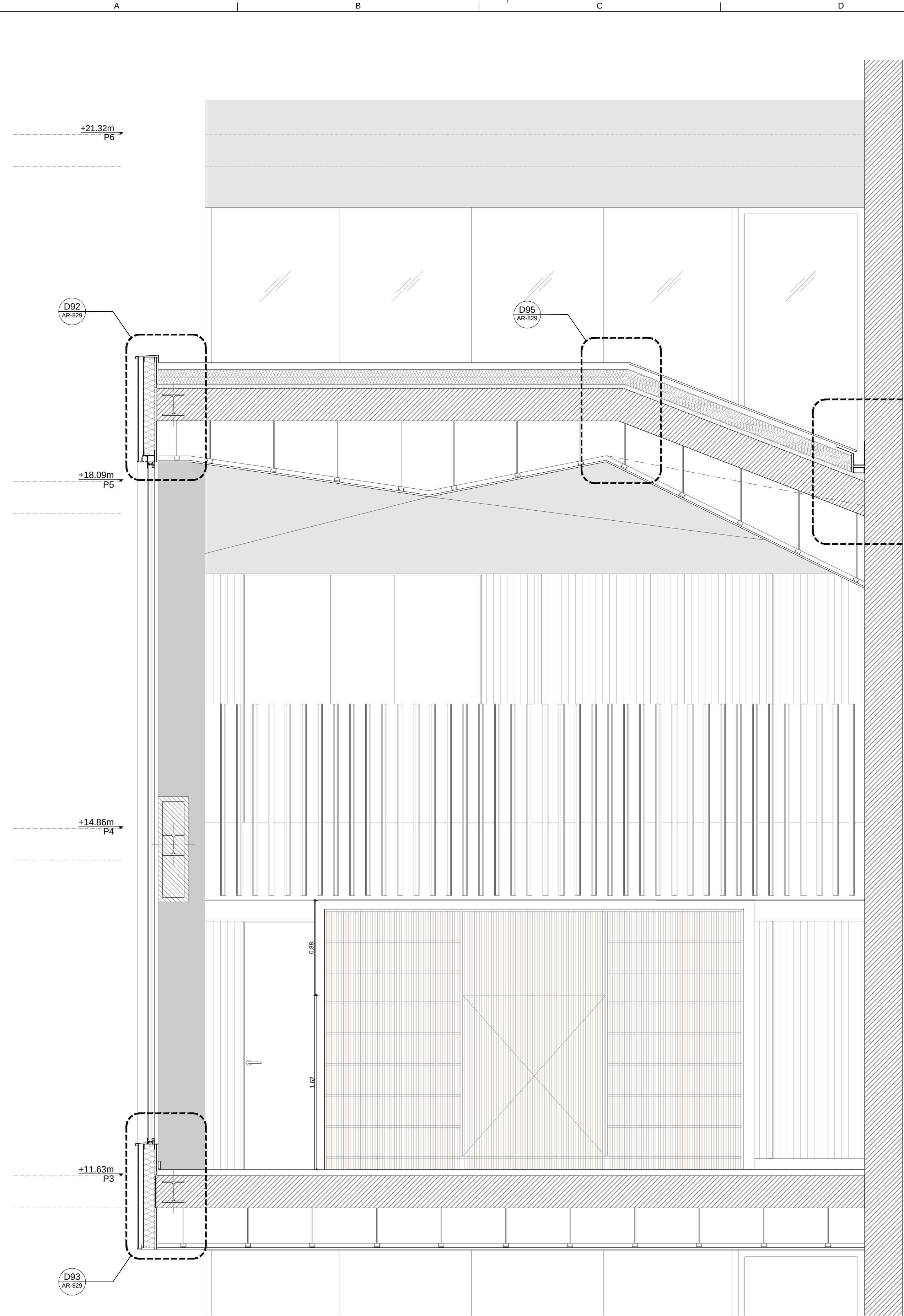
B7 Secció longitudinal
