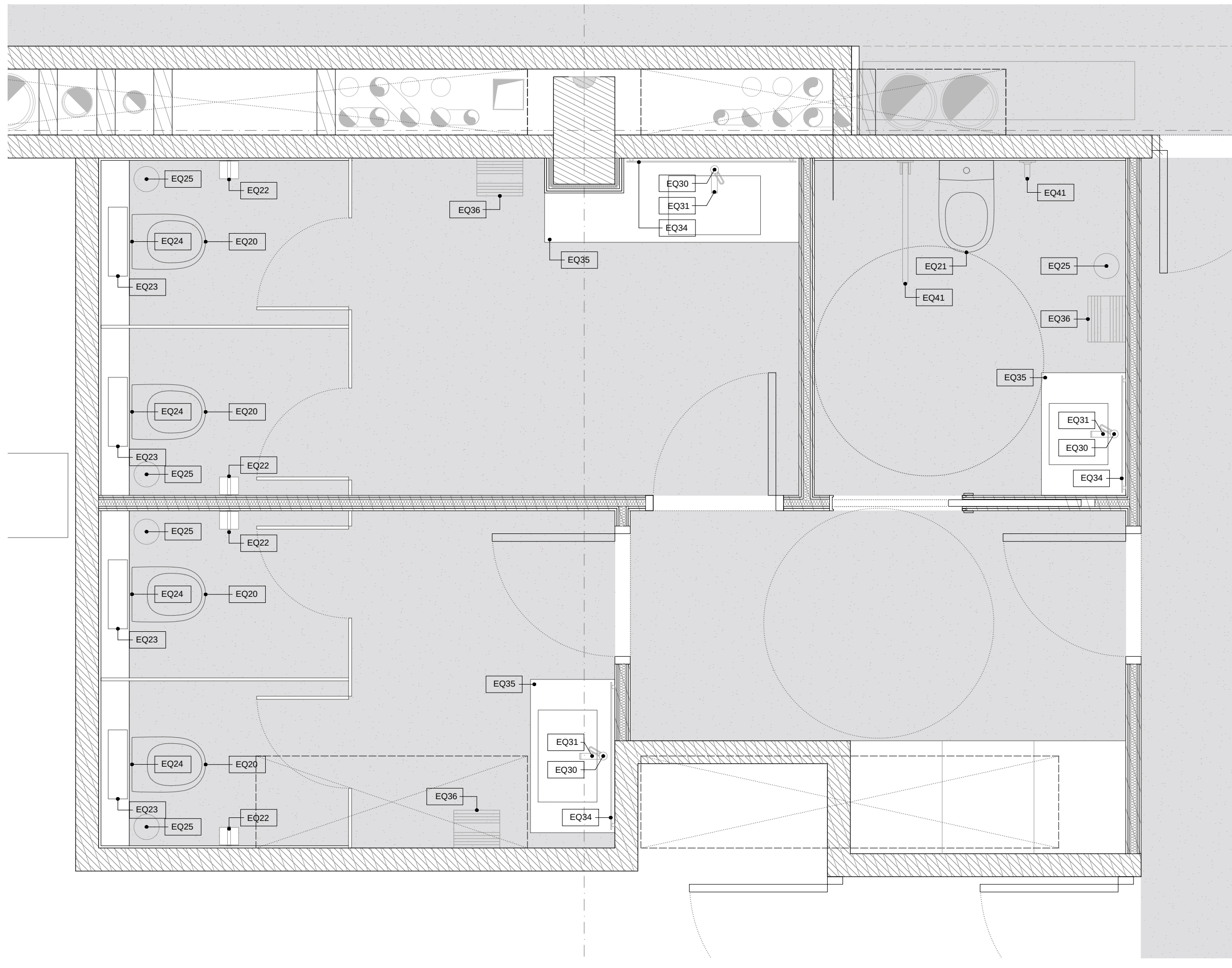
A5 Planta Equipaments Banys Comuns P01 A1 1:25 A3 1:50 0 25 50 75 100 150 200 250 cm
