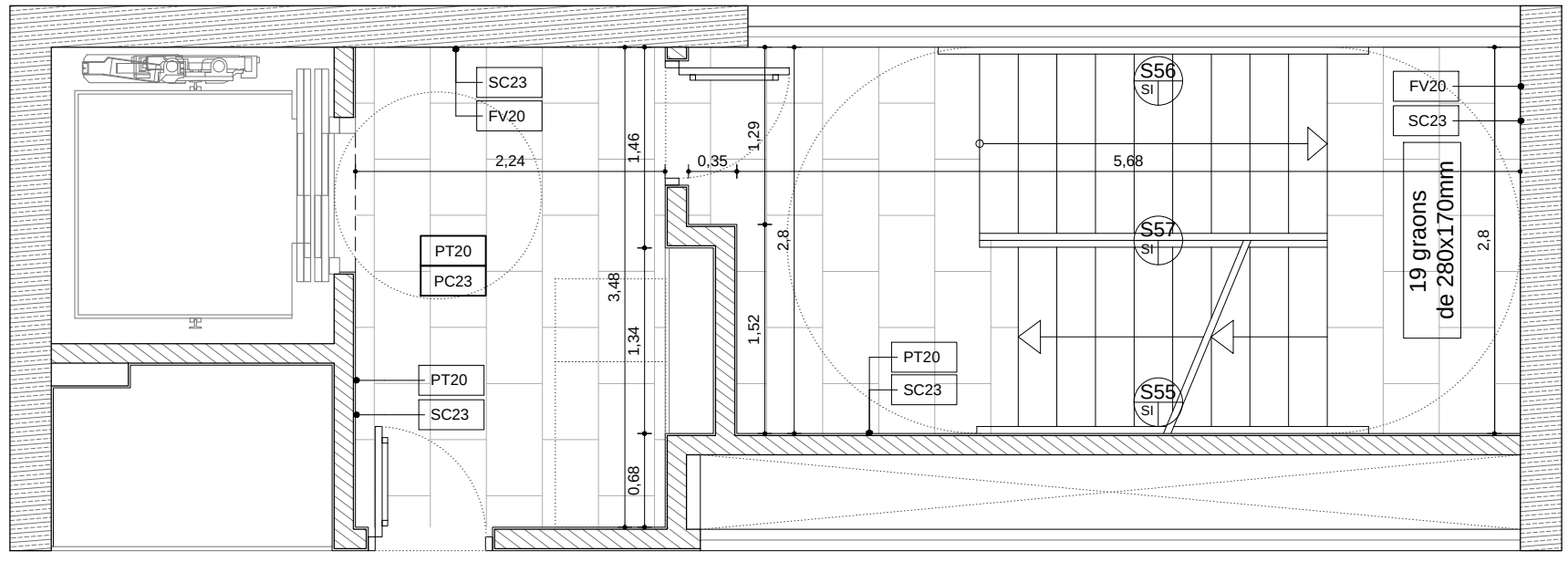
A5 Planta escala - P03-15
