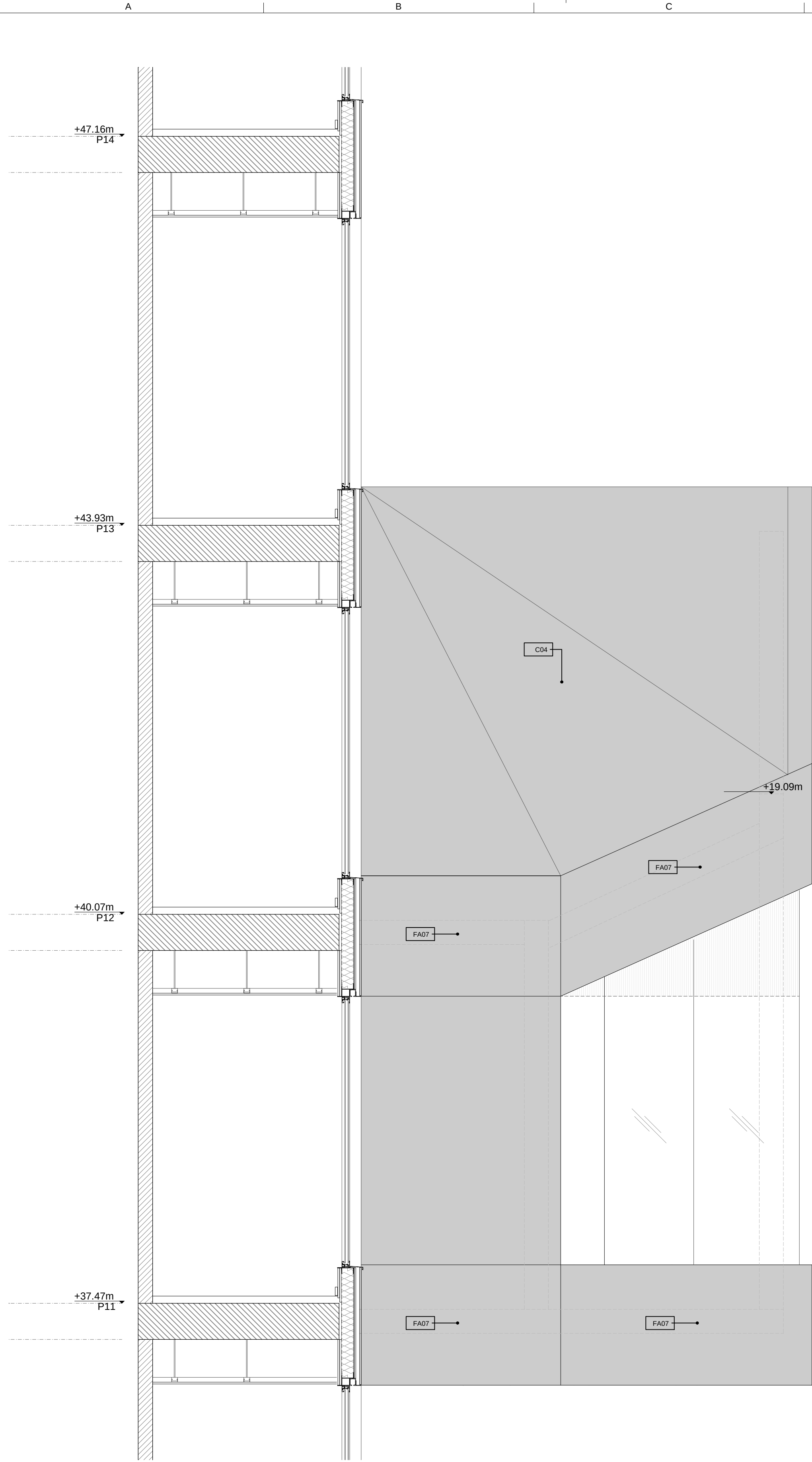
B7 Lateral exterior PP4 Oest
