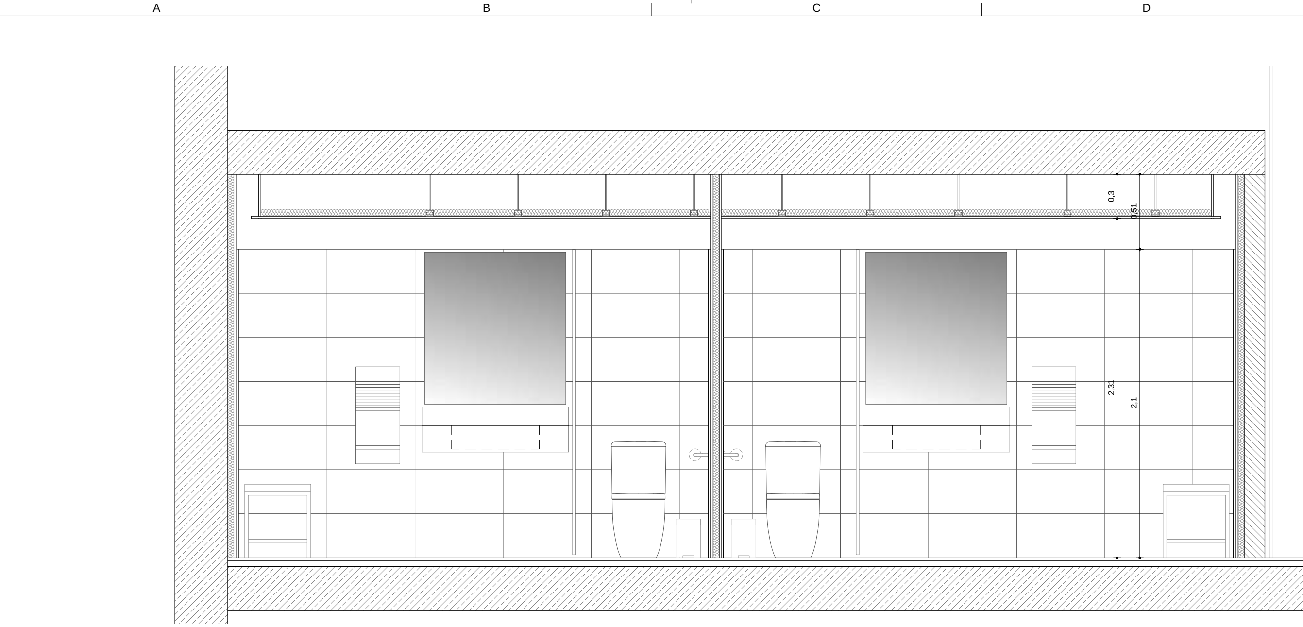
A3 Secció C
