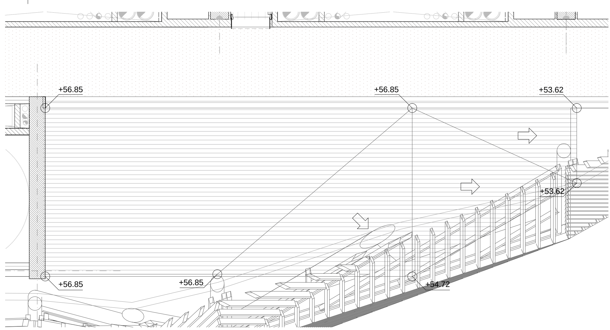
G5 Planta coberta
