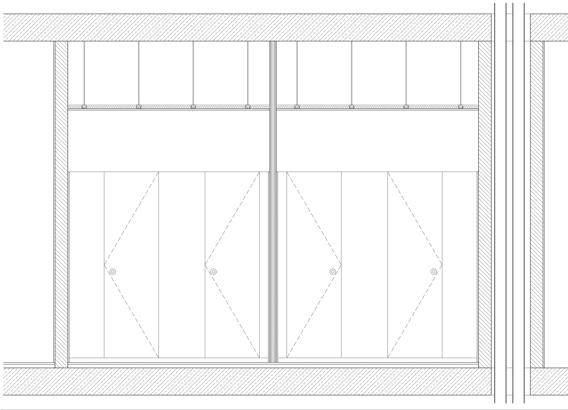
5F | Secció BB' A1 1:25 A3 1:50 0 25 50 75 100 150 200 250 cm
