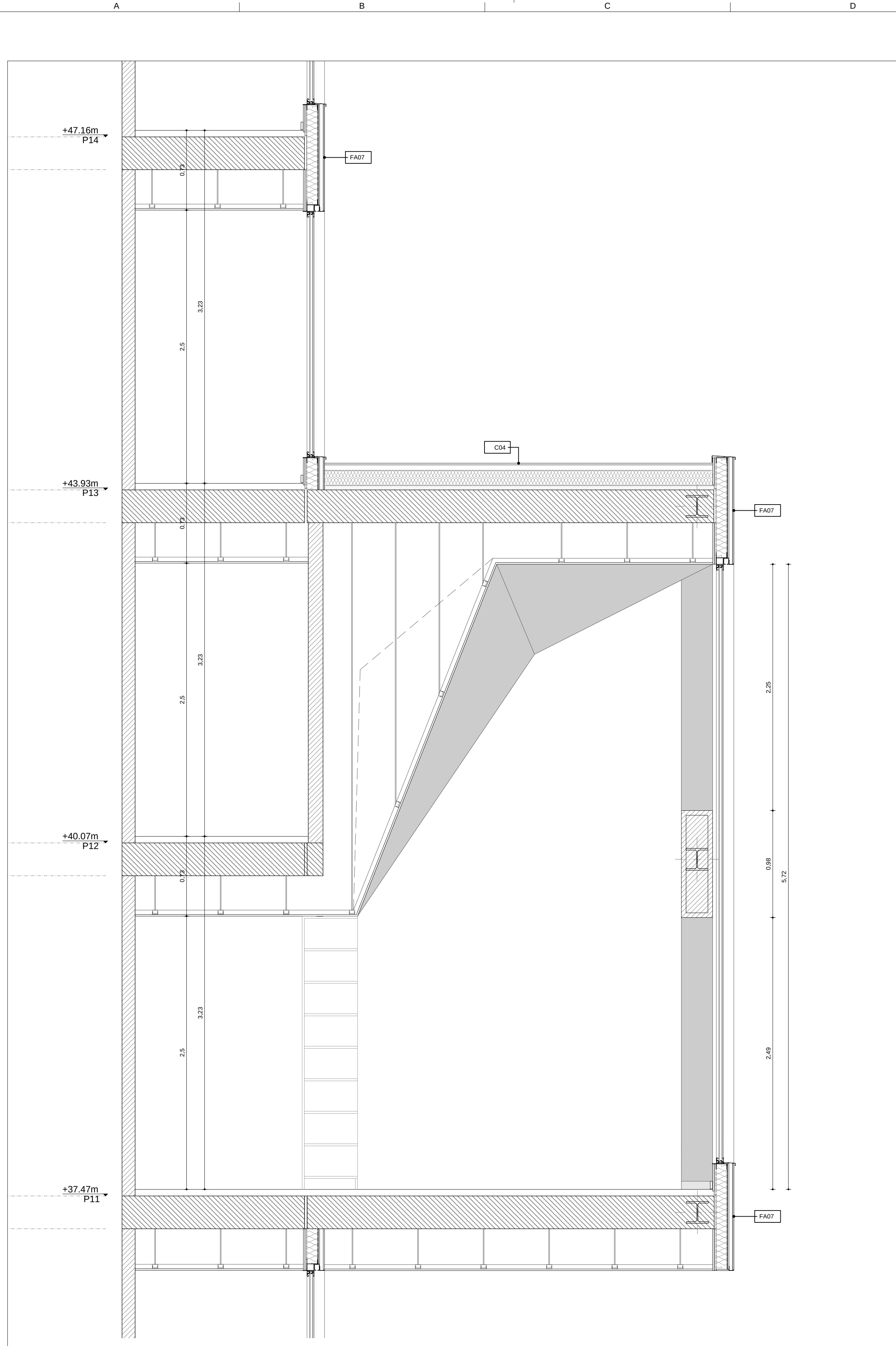
A7 Secció transversal A1 1:25 A3 1:50 0 25 50 75 100 150 200 250 cm
