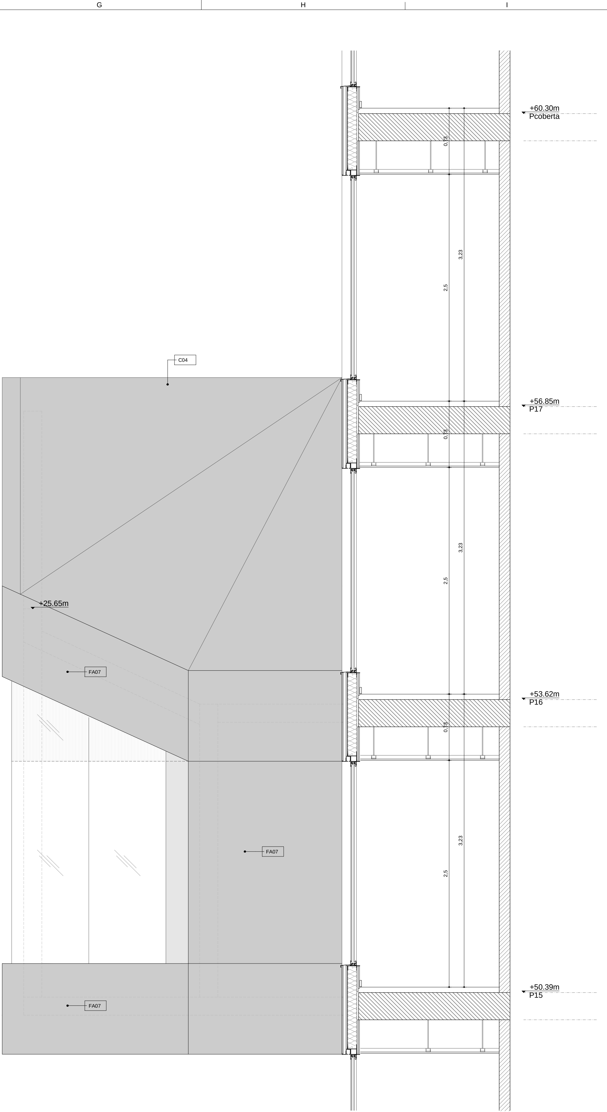
G7 Alçat transversal exterior
