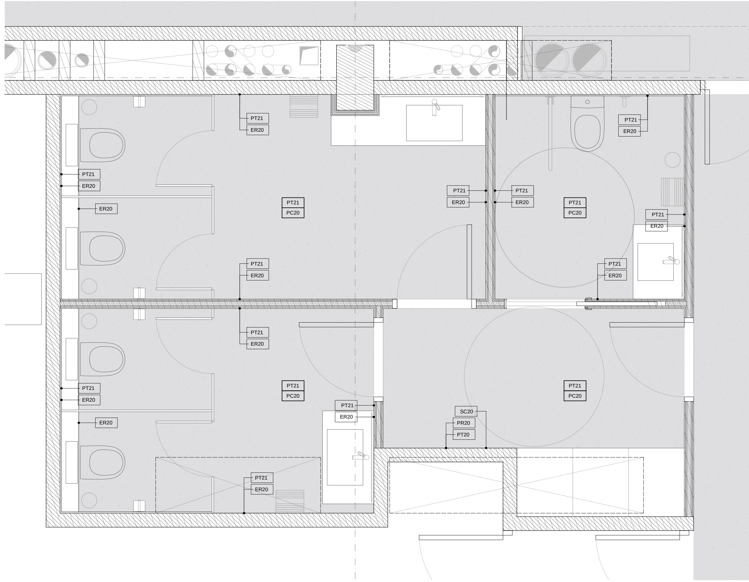
E5 | Planta Acabats Banys Comuns P01 A1 1:25 A3 1:50 0 25 50 75 100 150 200 250 cm
