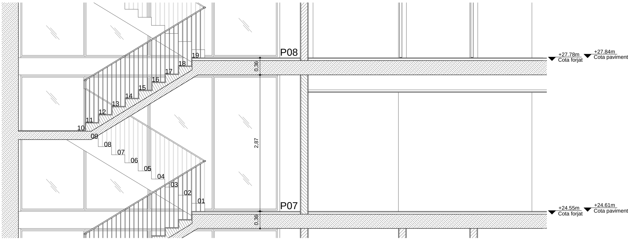
E3 Secció escala P07 i P15
