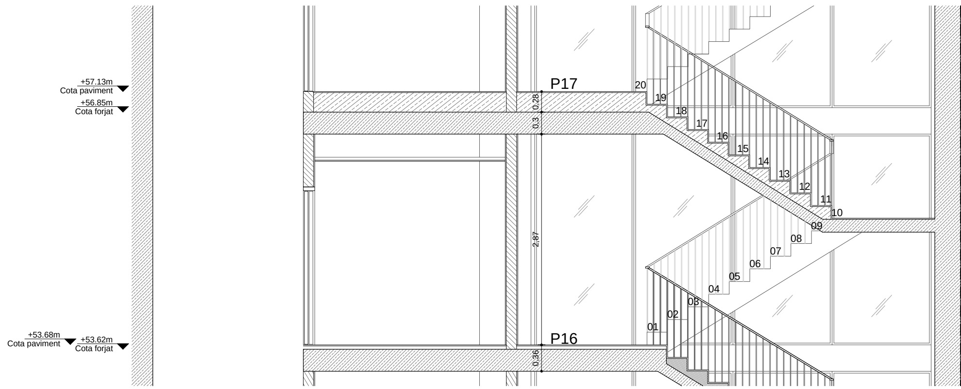
D5 Secció escala - P16
