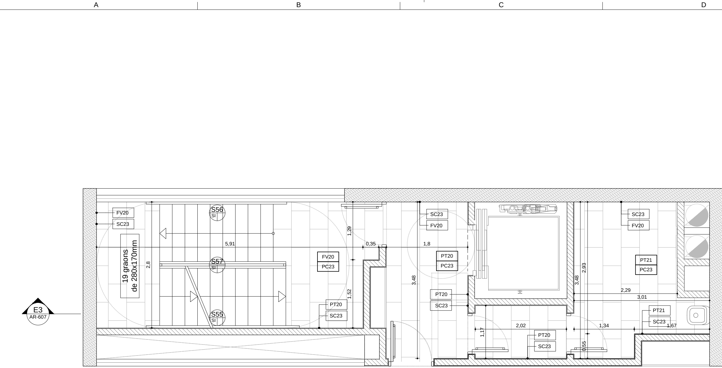
A3 Planta escala - P02
