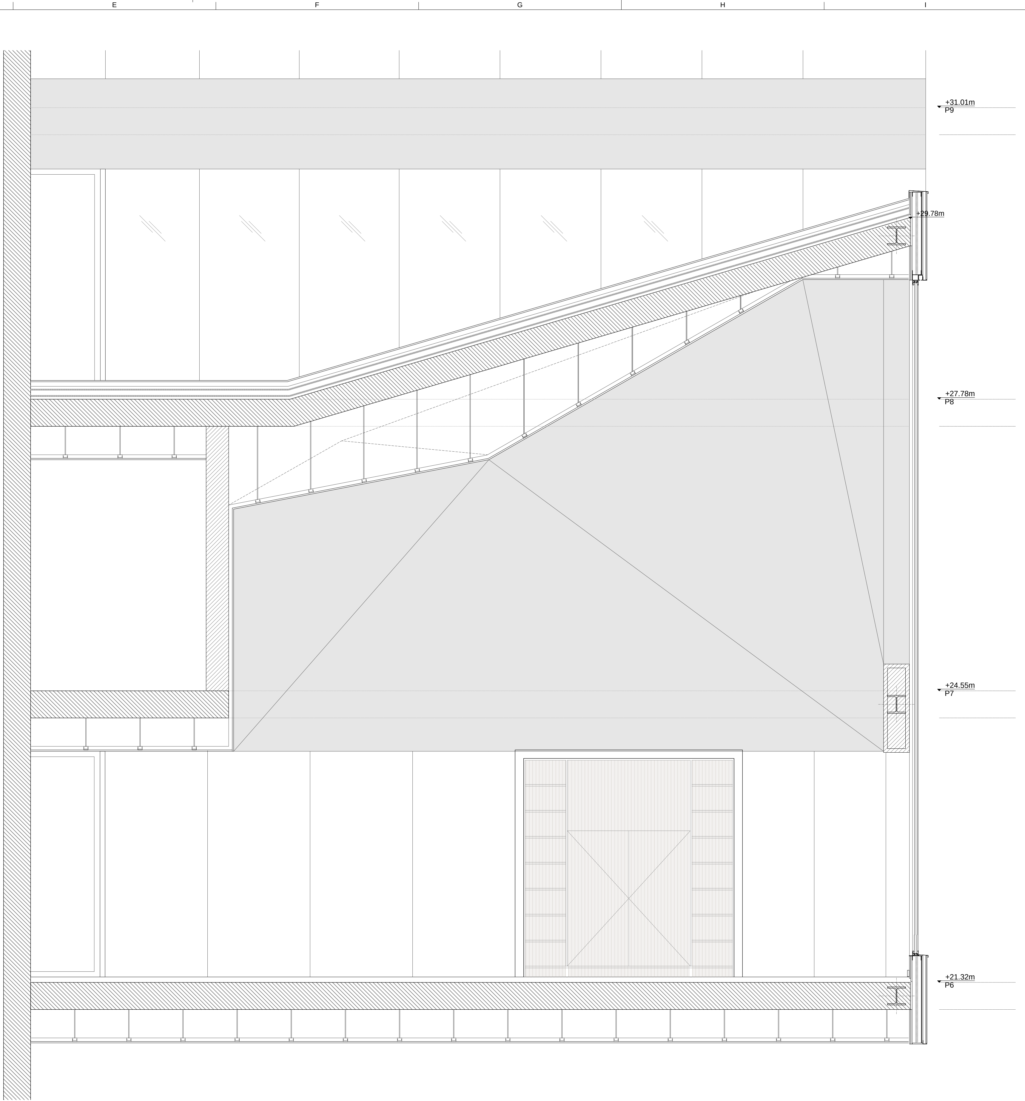
E7 Alçat longitudinal interior
