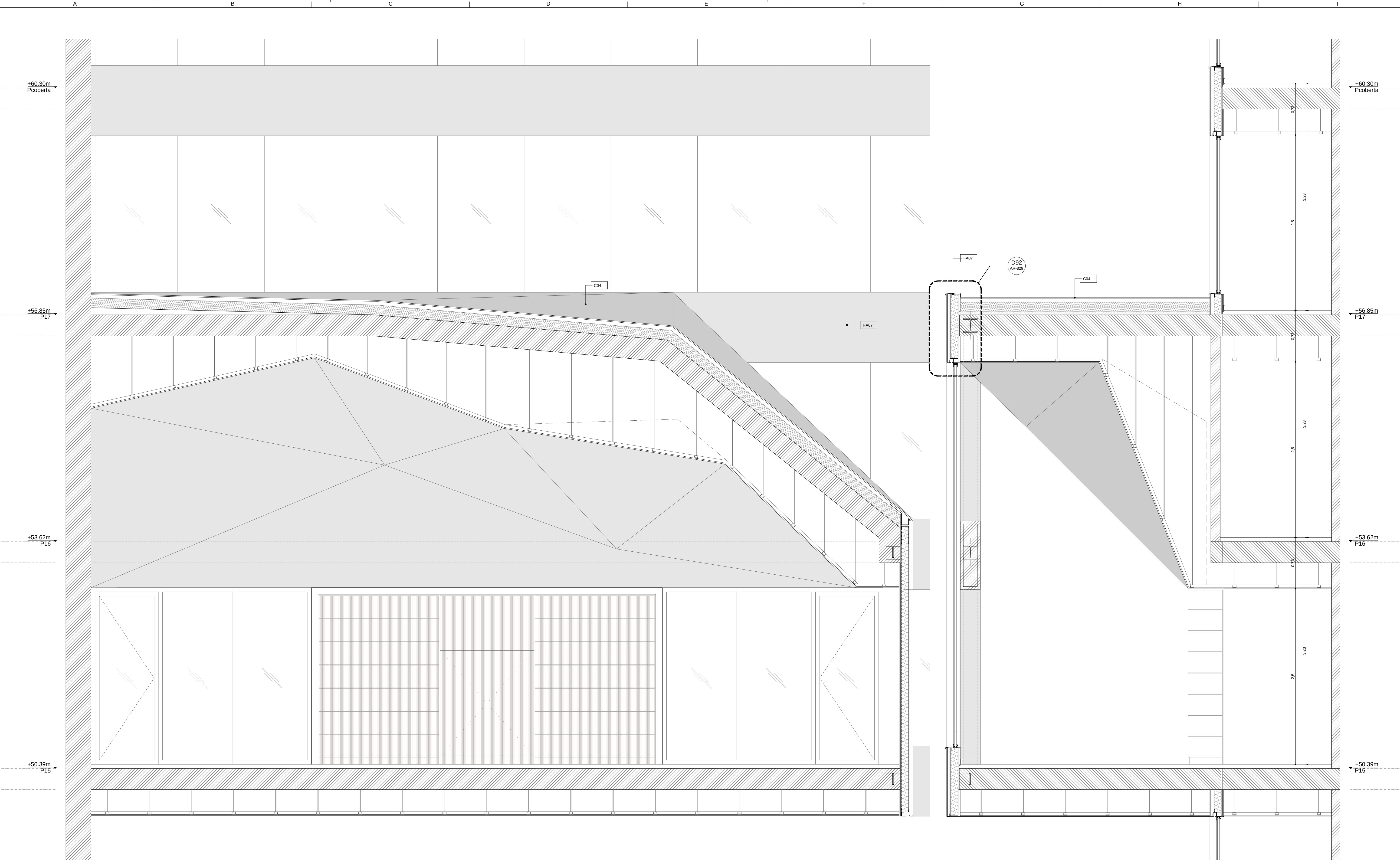
A7 Secció longitudinal
