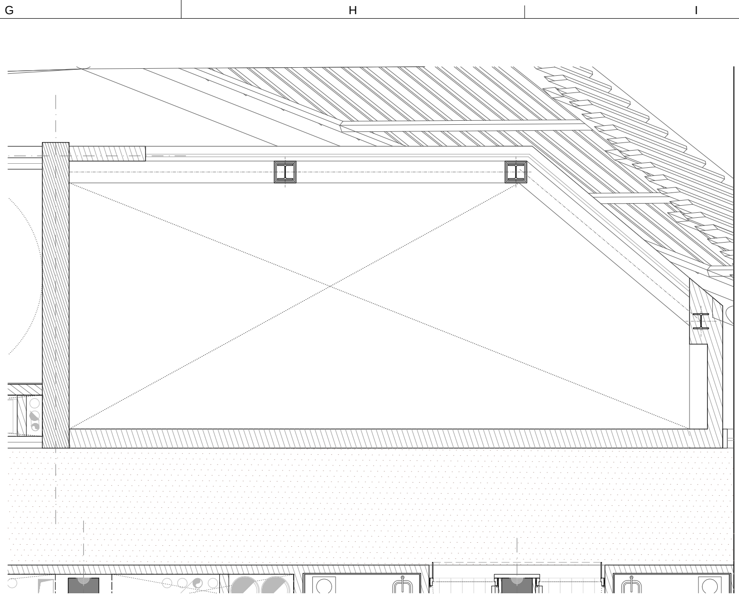
F3 Planta doble alçada
