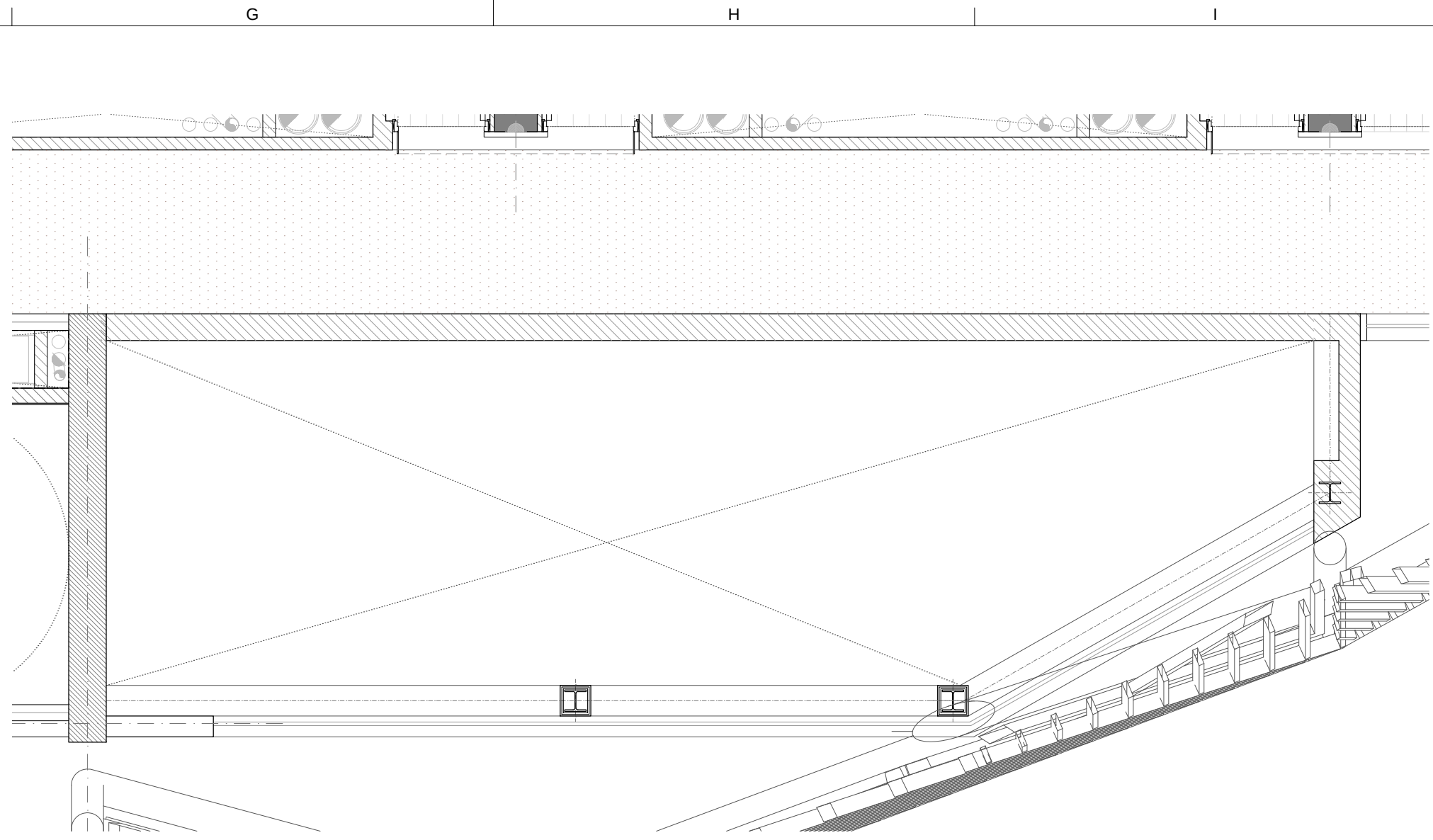
G3 Planta doble alçada
