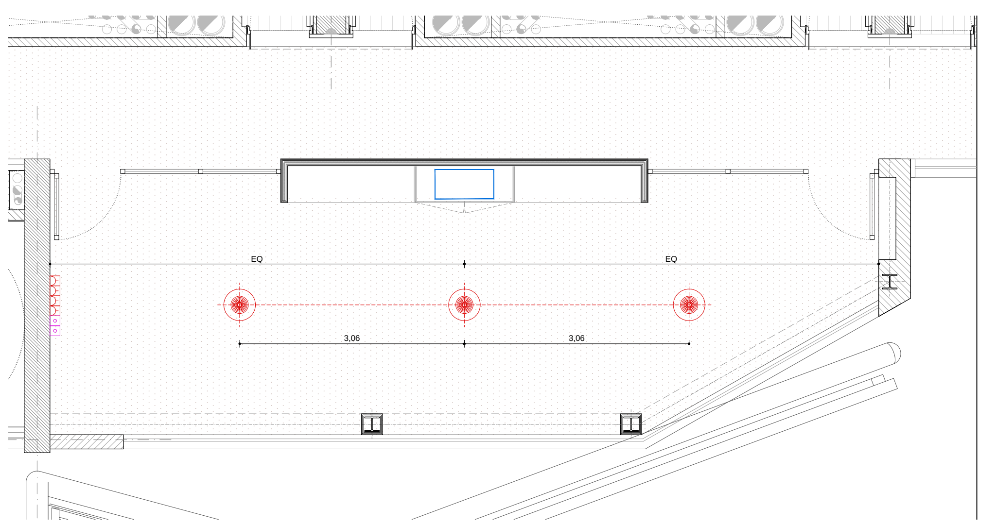
G7 Planta il·luminació
