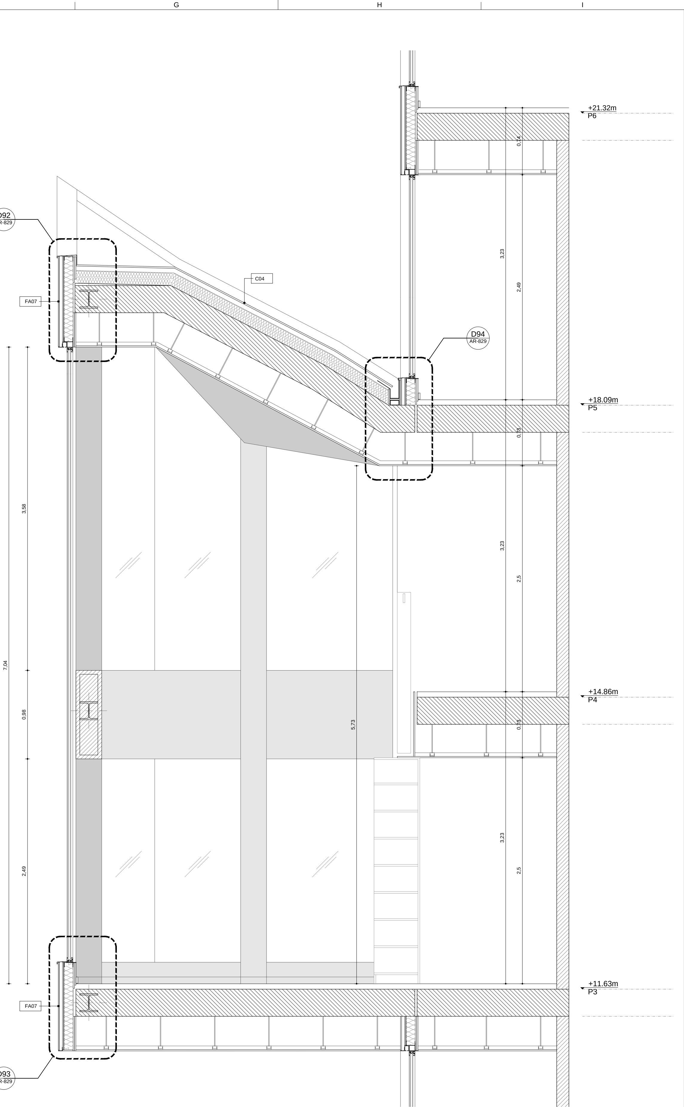
F7 Secció transversal
