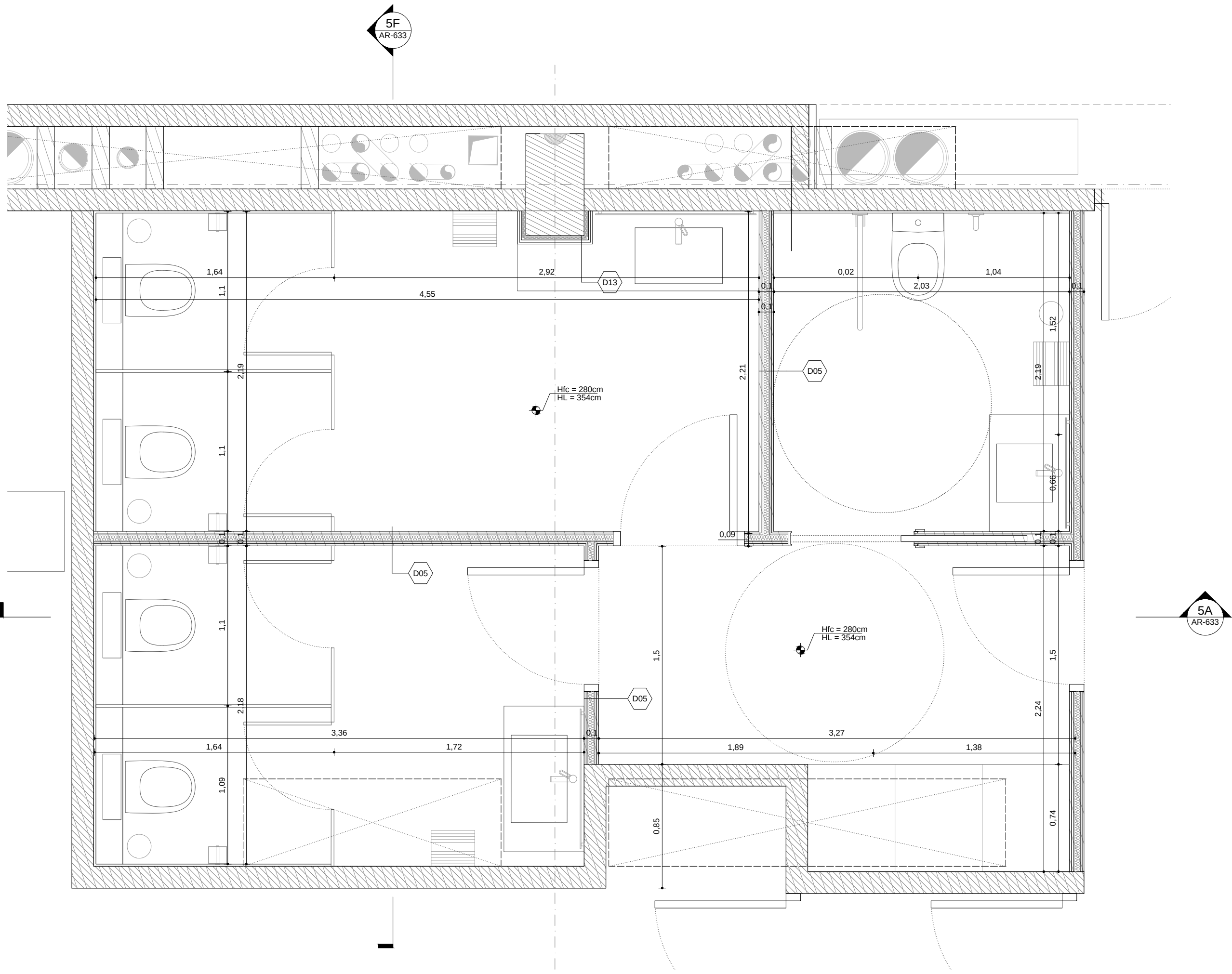
A5 | Planta Acotacions Banys Comuns P01 A1 1:25 A3 1:50 0 25 50 75 100 150 200 250 cm
