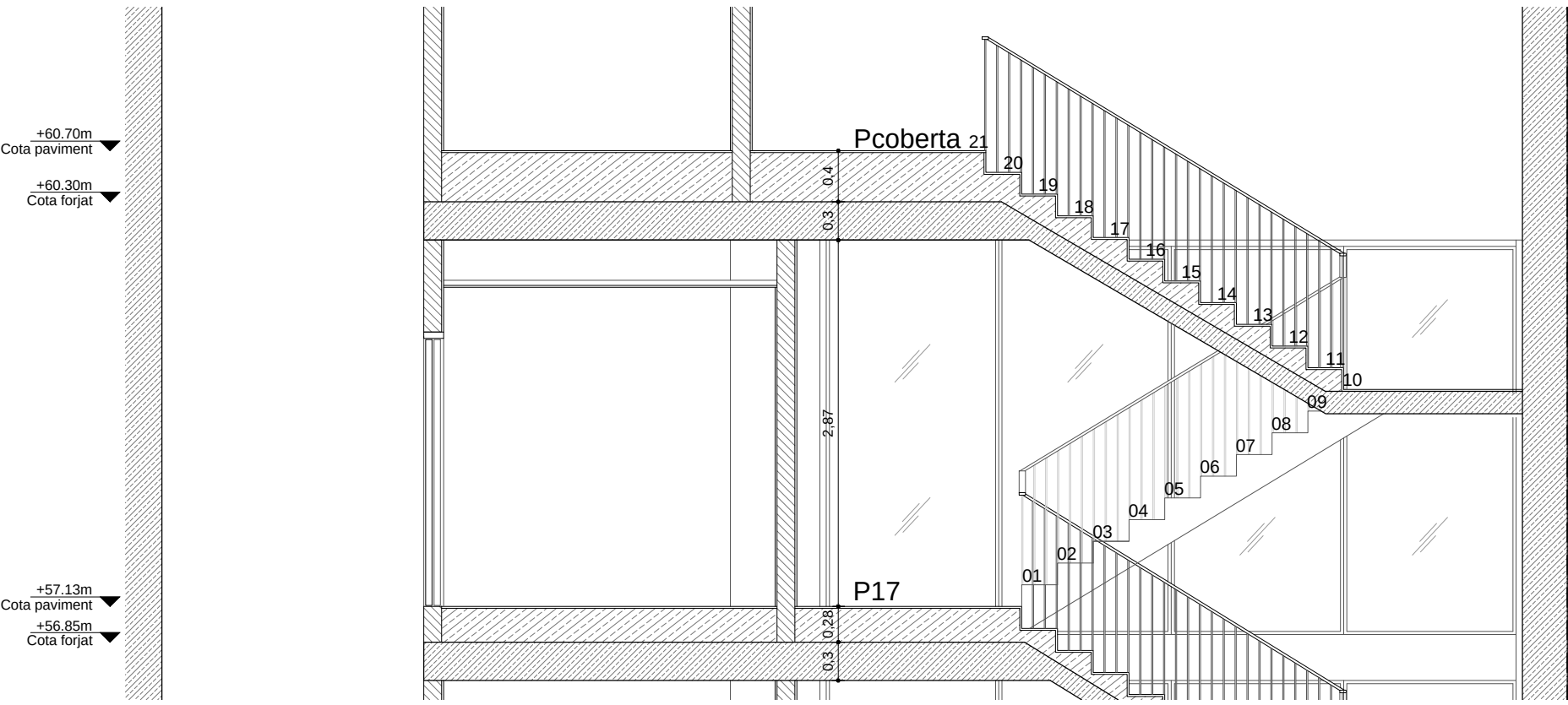
D3 Secció escala P17
