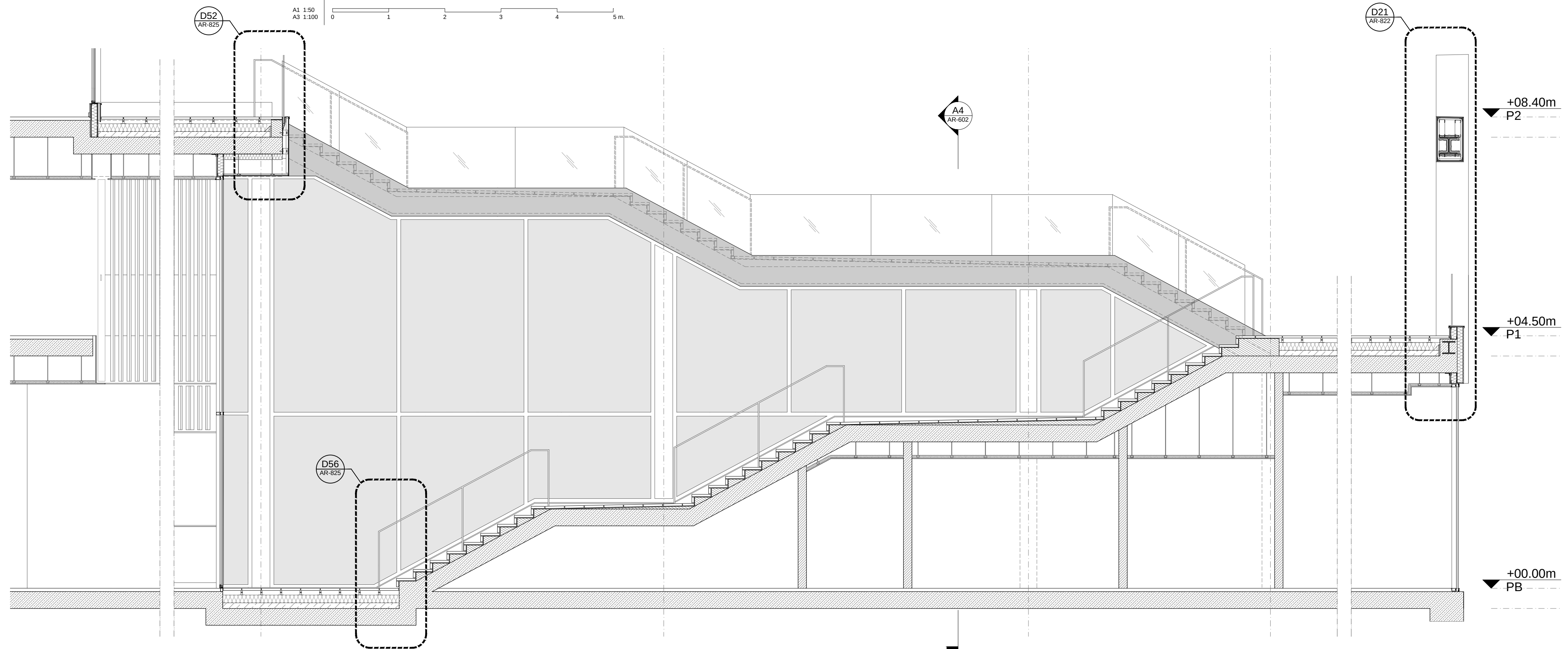
C7 | Secció Tram 1 - P00 a P01
