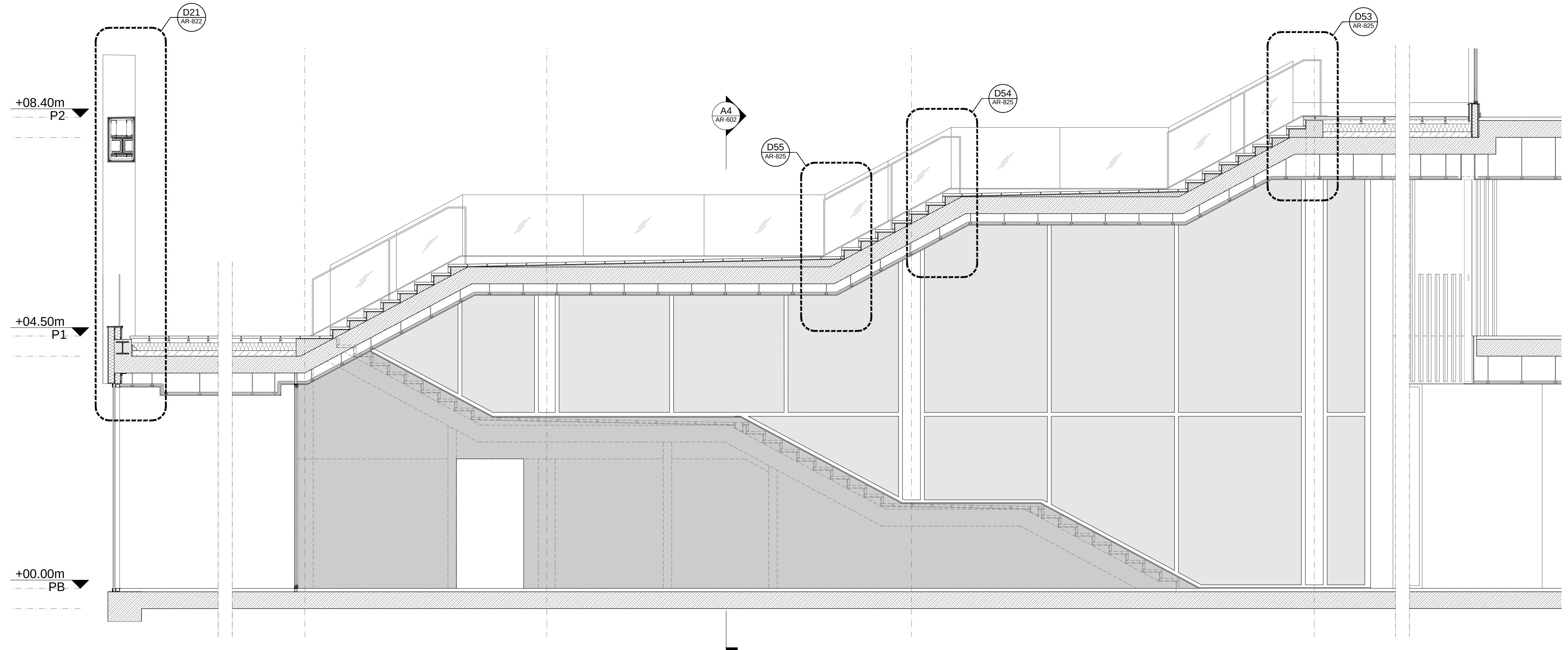
C4 | Secció Tram 2 - P01 a P02
