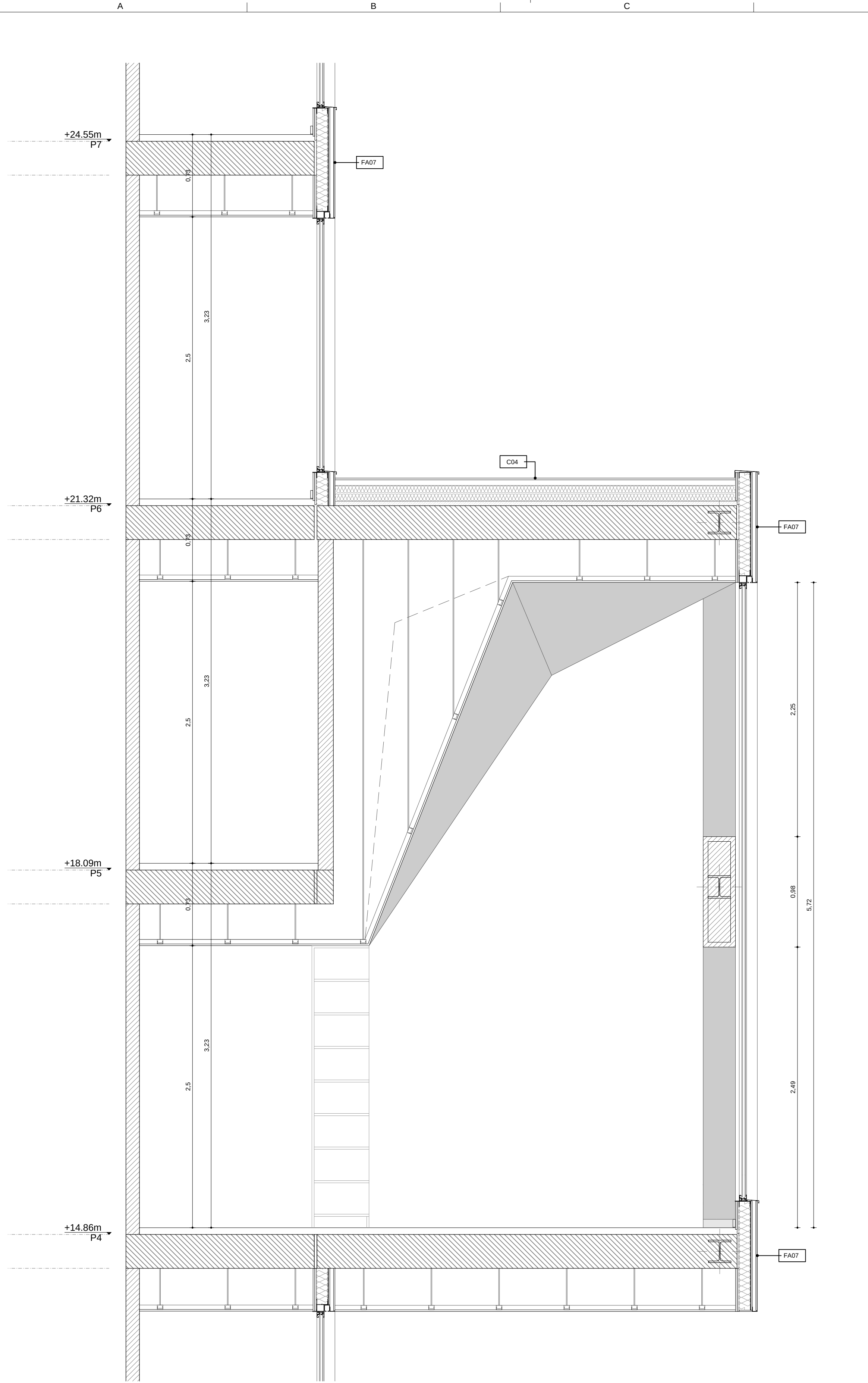
A7 Secció transversal
