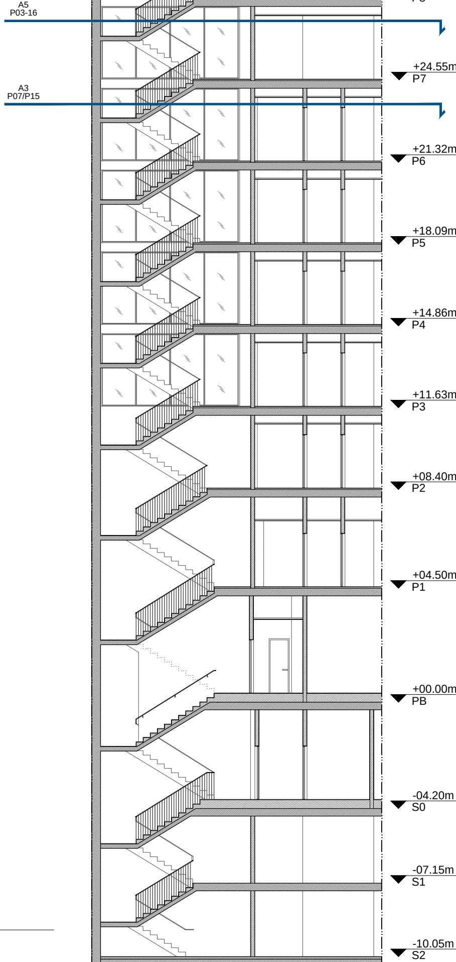
H7 Secció General - ALA EST
