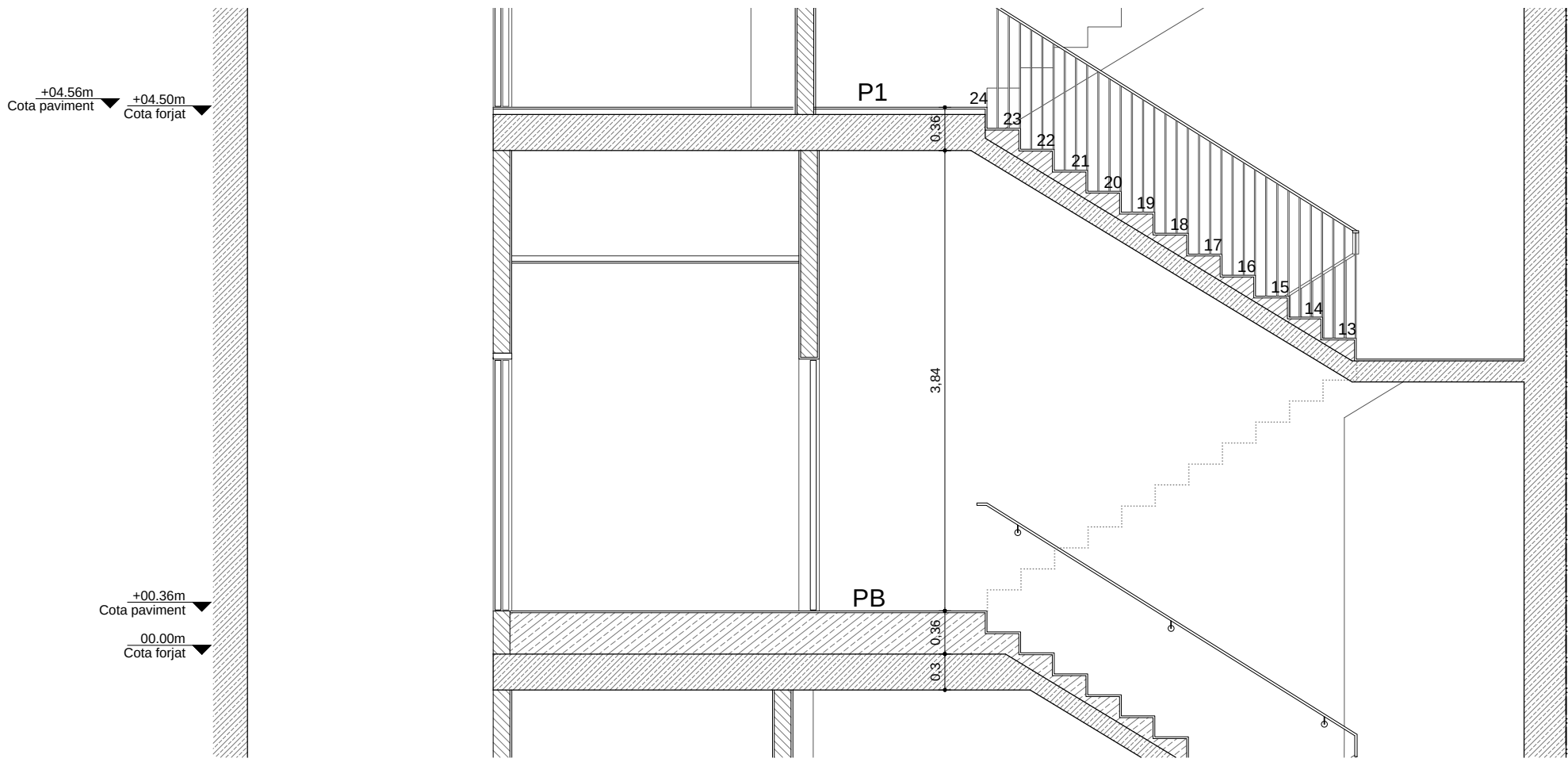
D3 Secció escala - PB
