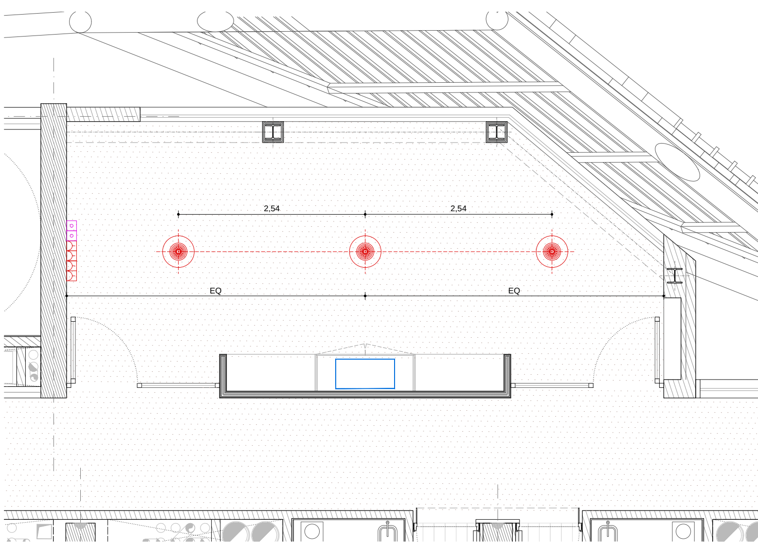
F7 Planta il·luminació
