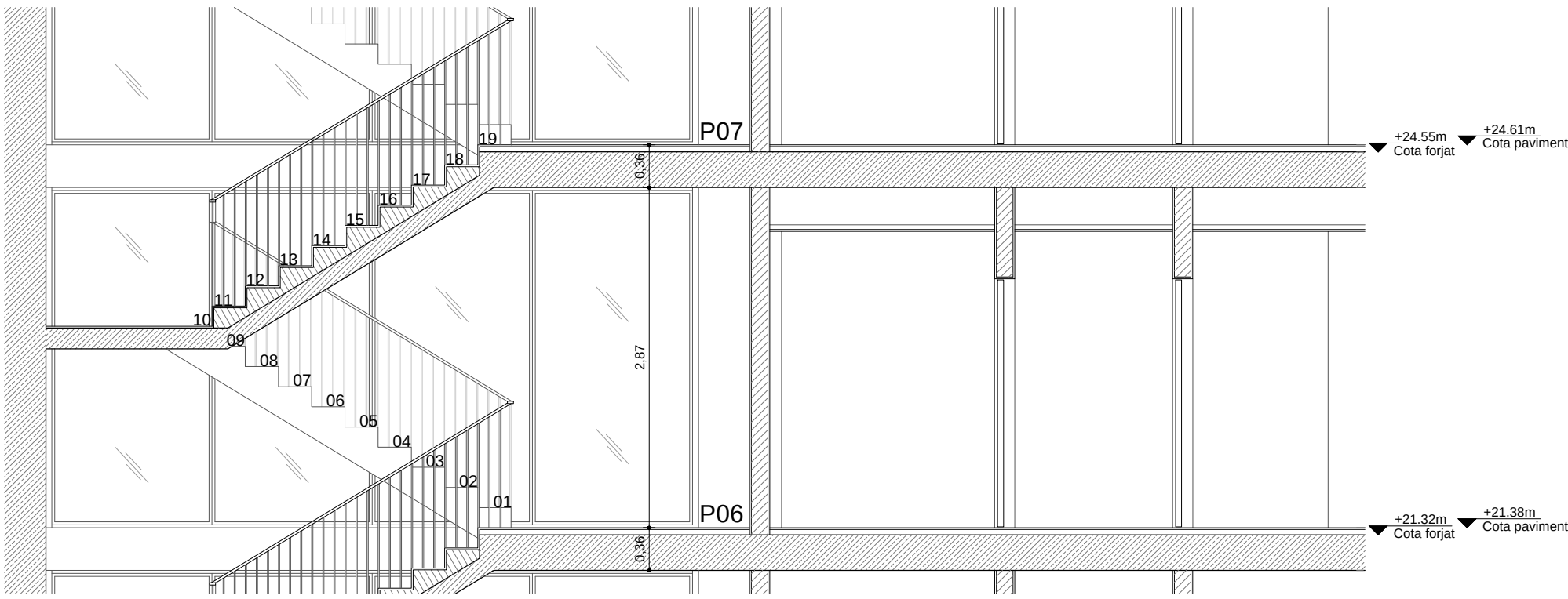
E5 Secció escala - P03-16
