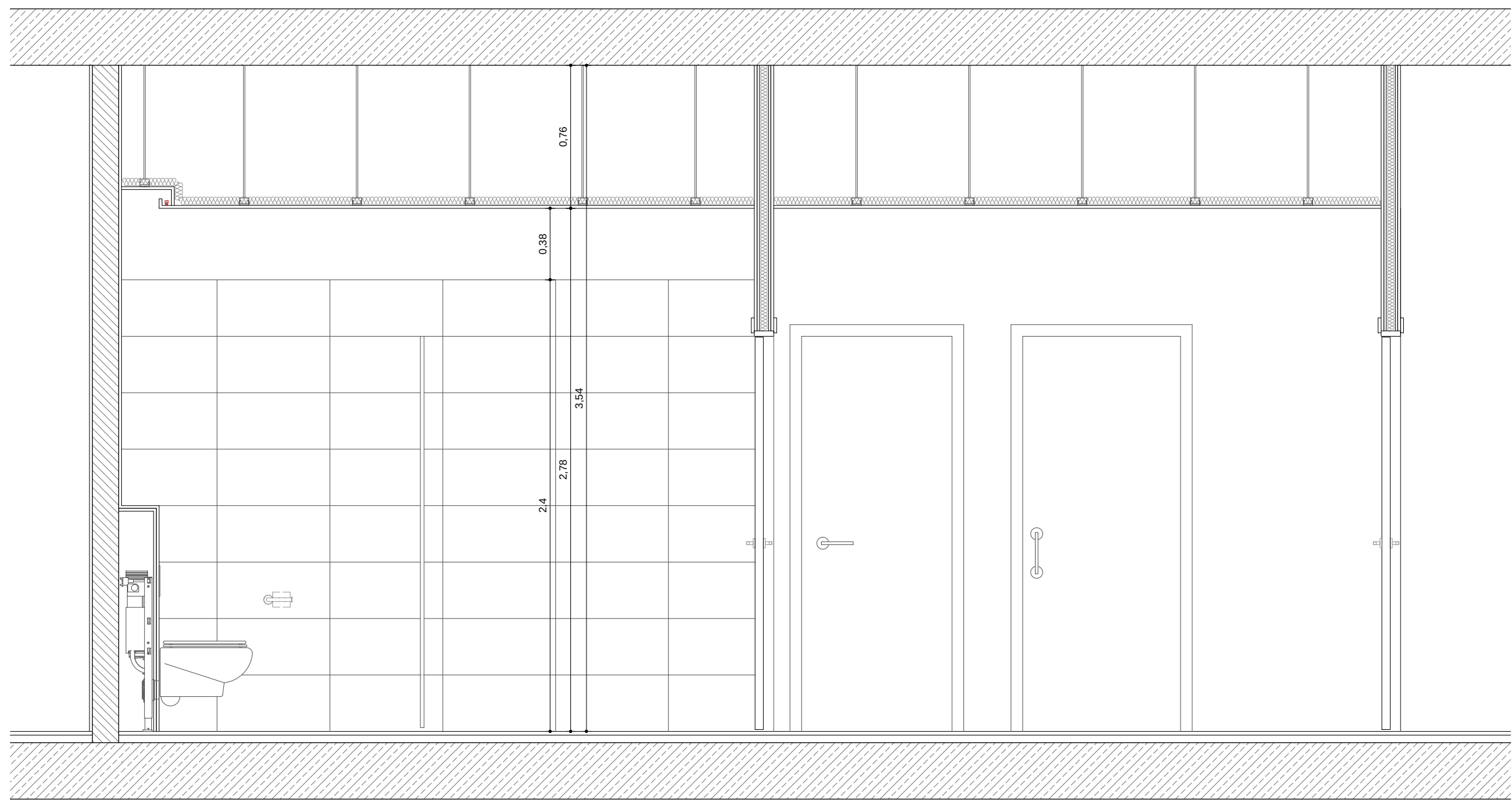
5A | Secció AA' A1 1:25 A3 1:50 0 25 50 75 100 150 200 250 cm
