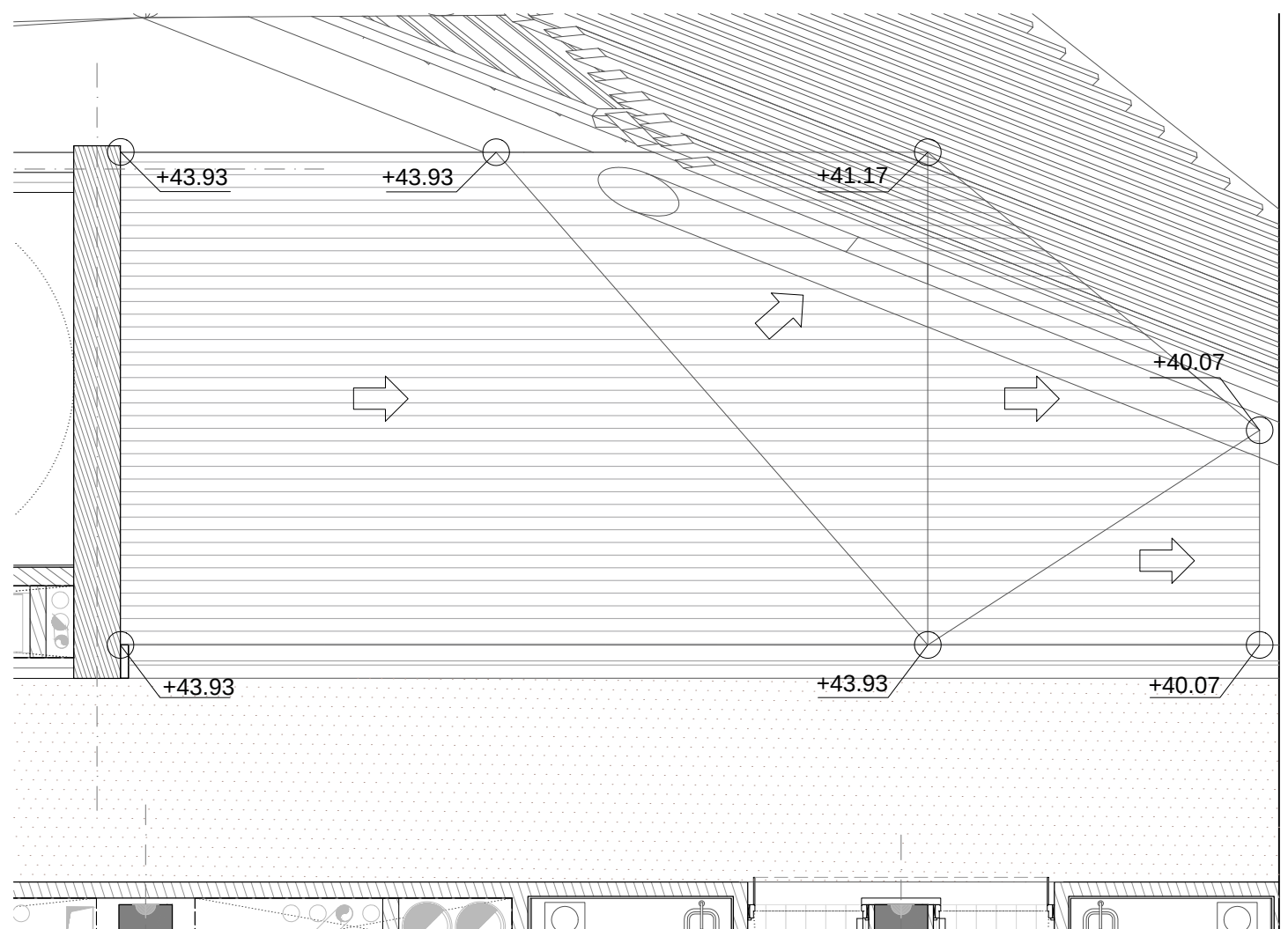
F5 Planta coberta
