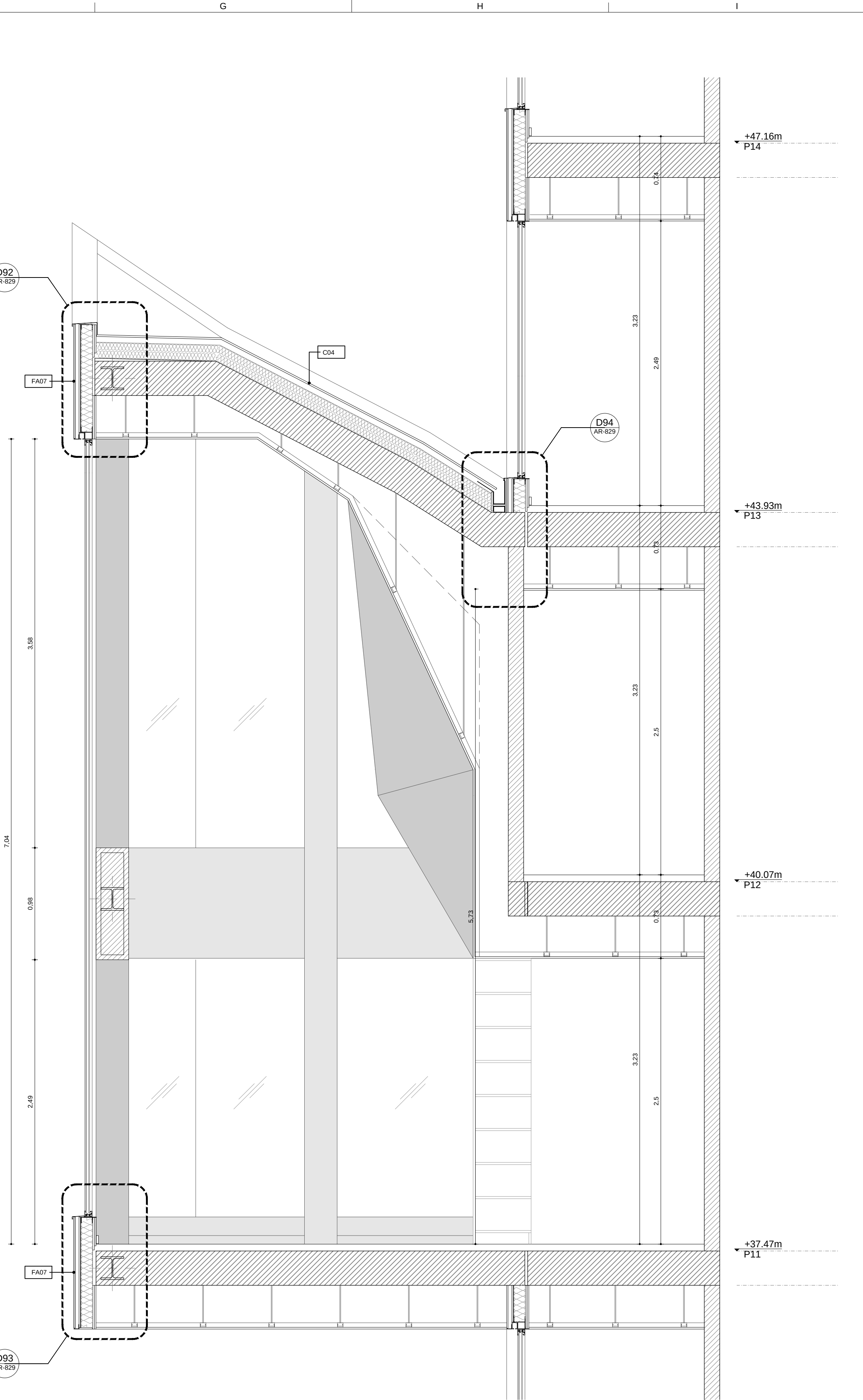
F7 Secció transversal A1 1:50 A3 1:100 0 1 2 3 4 5 m.
