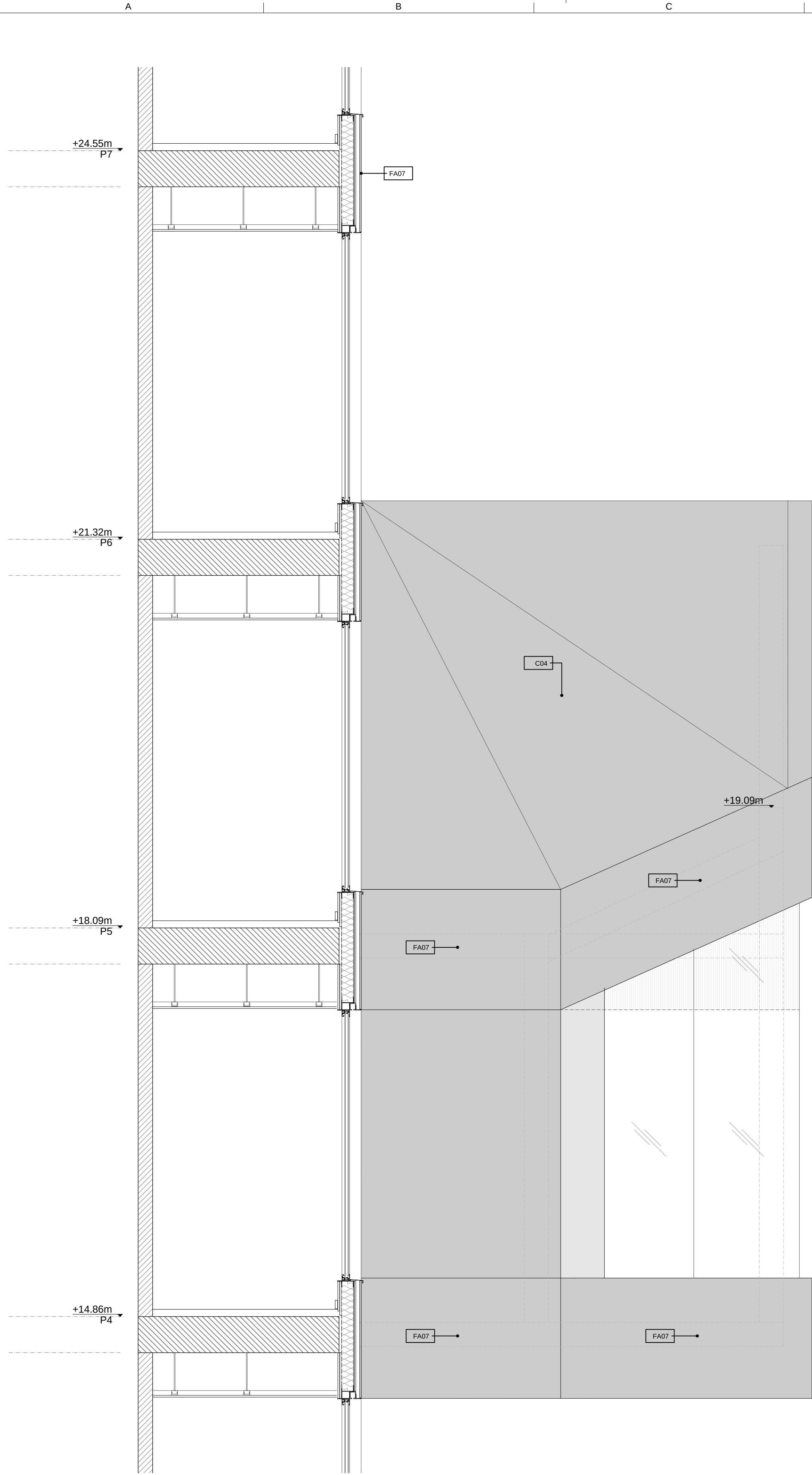
B7 Lateral exterior PP4 Oest A1 1:25 A3 1:50 0 25 50 75 100 150 200 250 cm
