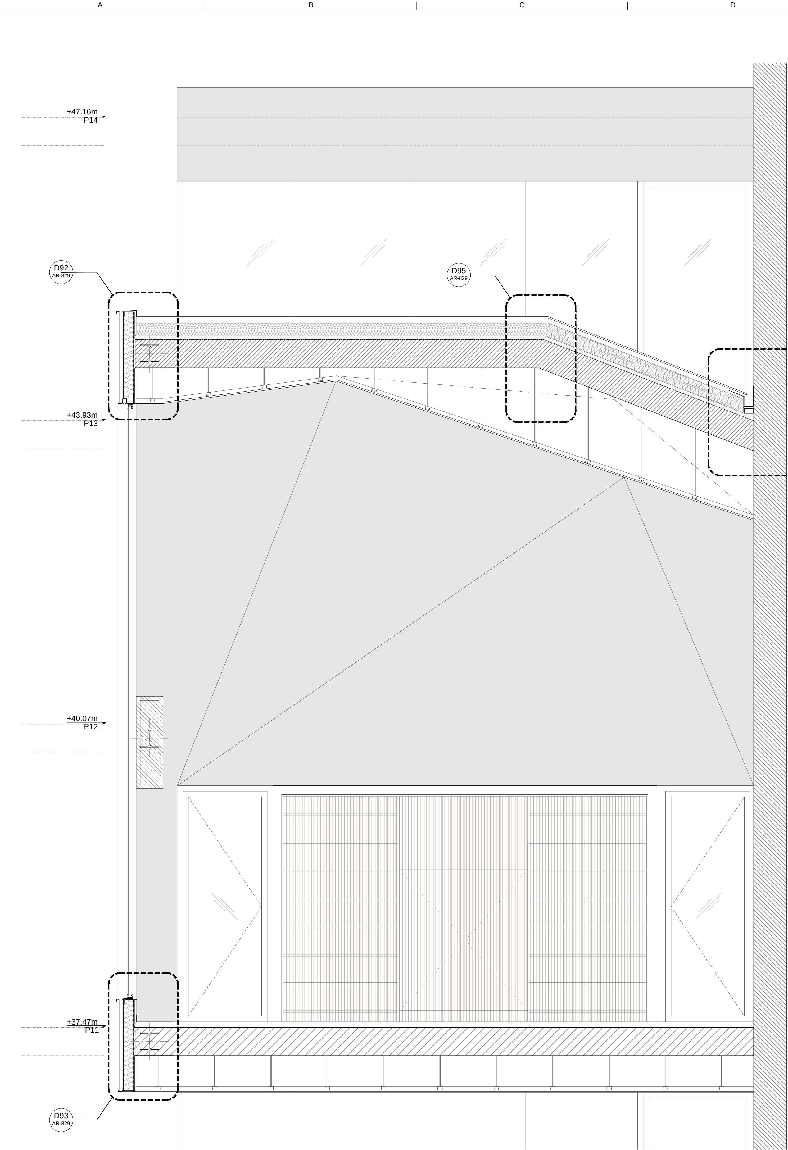
B7 Secció longitudinal A1 1:25 A3 1:50 0 25 50 75 100 150 200 250 cm
