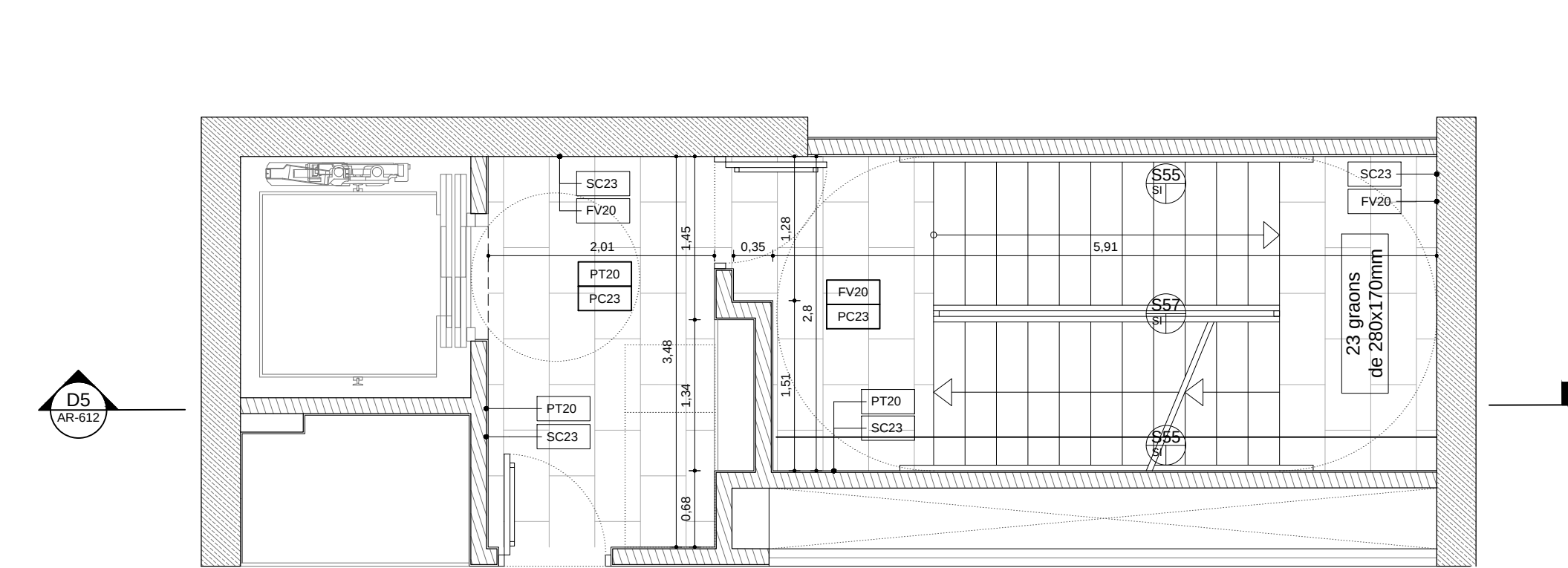
A5 Planta escala - P01
