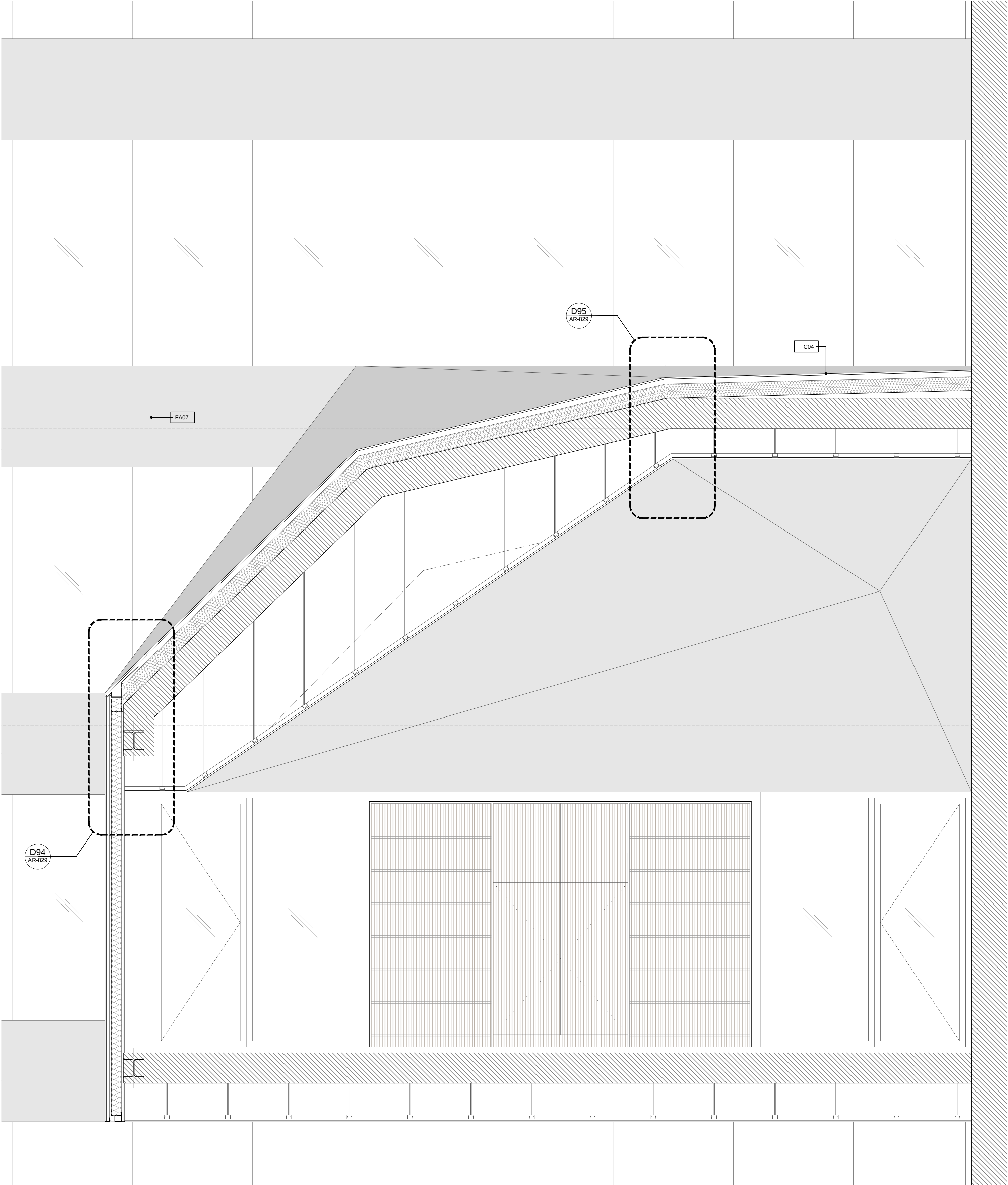
E7 Secció longitudinal A1 1:50 A3 1:100 0 1 2 3 4 5 m
