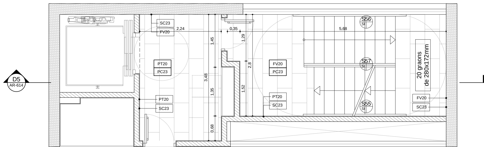
A5 Planta escala - P16
