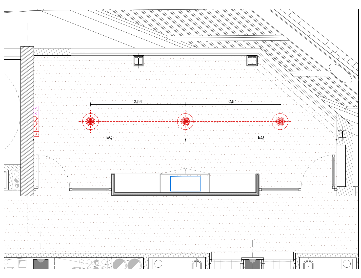
F7 Planta il·luminació
