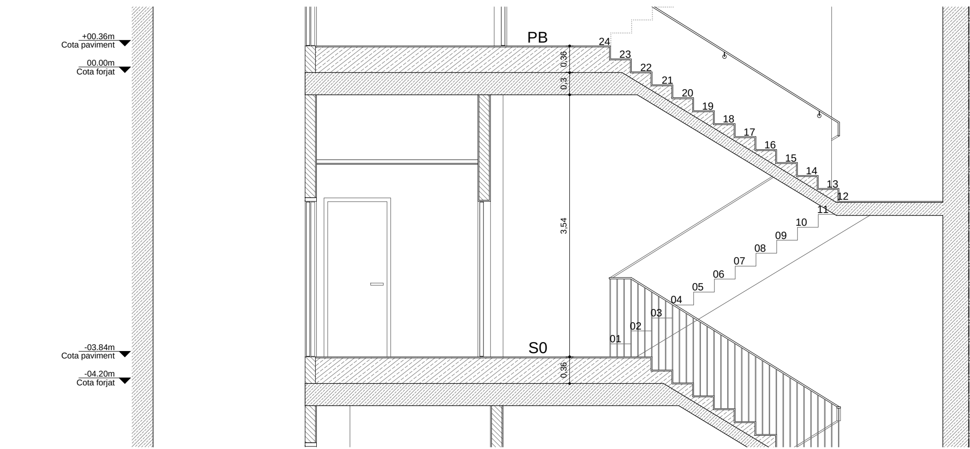
D5 Secció escala - Ps0
