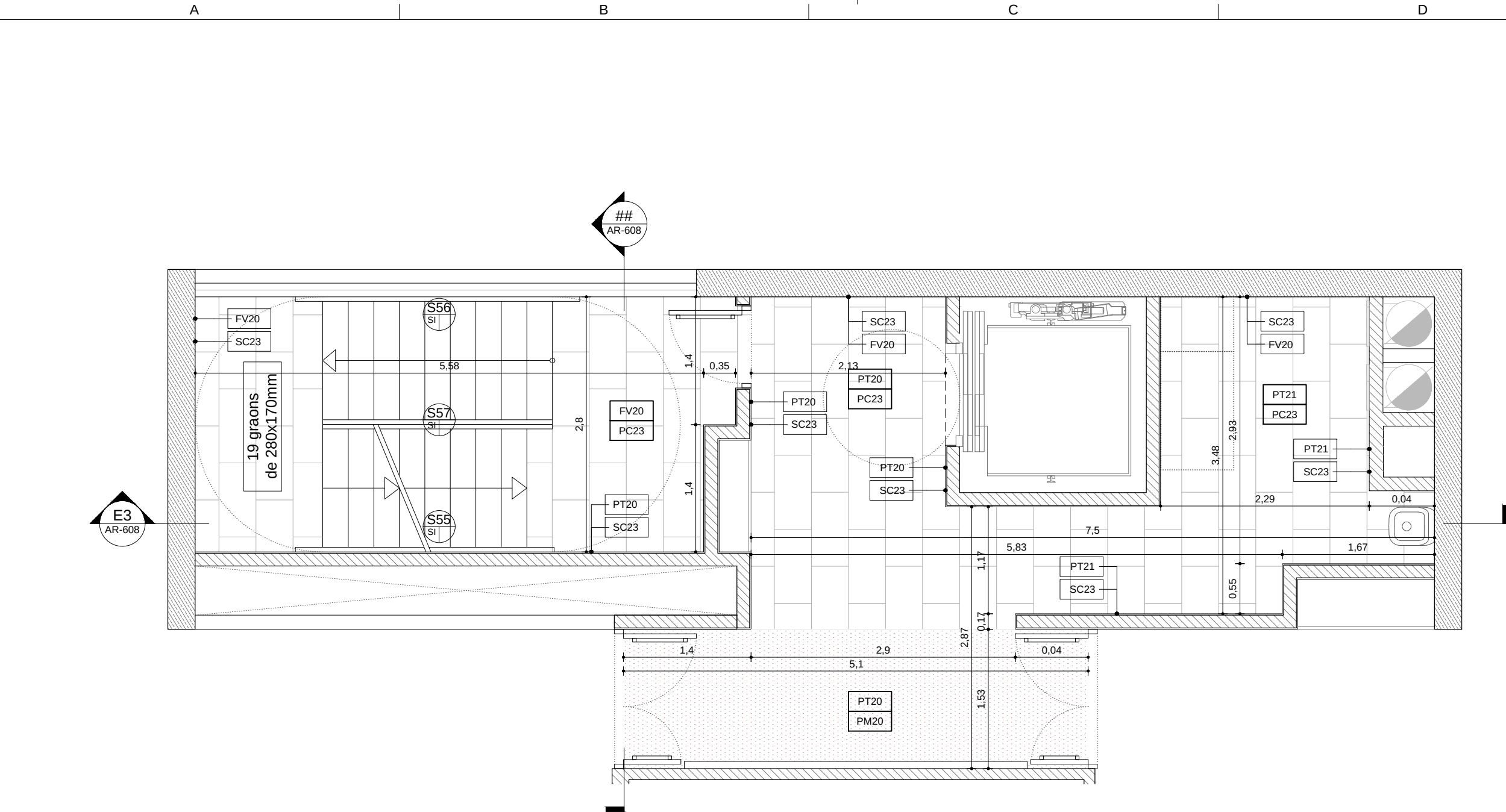
A3 Planta escala - P07 i P15
