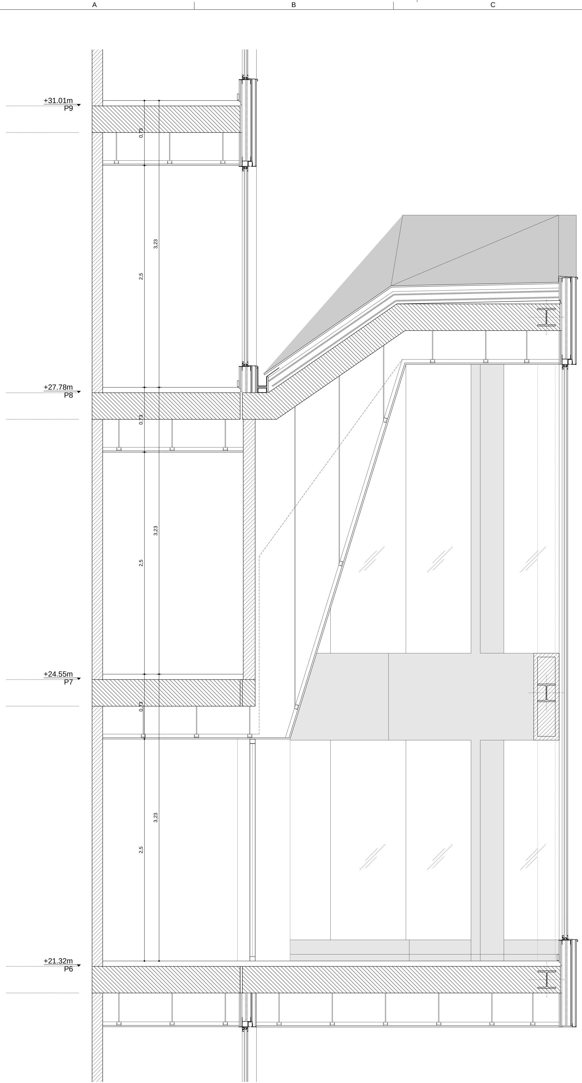
A7 Secció transversal
